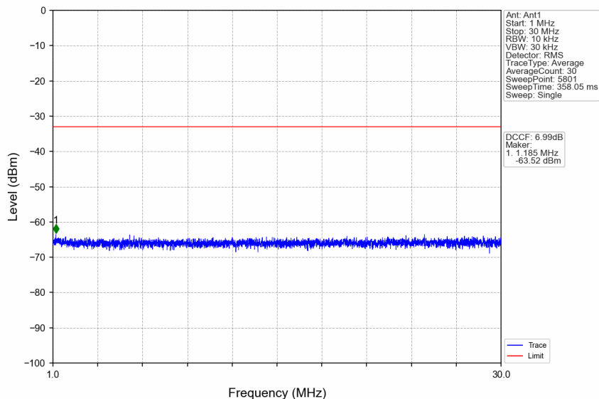
n38_30kHz_SISO_NTNV_30MHz_CP-OFDM QPSK_2595MHz_Edge_1RB_Left
