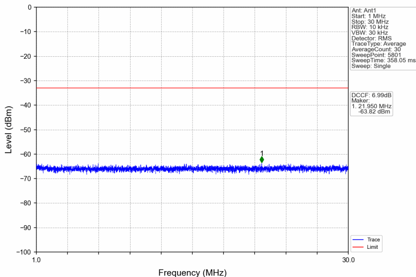
n38_30kHz_SISO_NTNV_40MHz_DFT-s-OFDM PI/2 BPSK_2595MHz_Edge_1RB_Left
