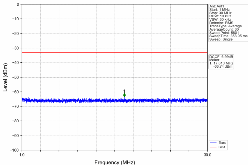
n38_30kHz_SISO_NTNV_40MHz_DFT-s-OFDM QPSK_2590MHz_Edge_1RB_Left
