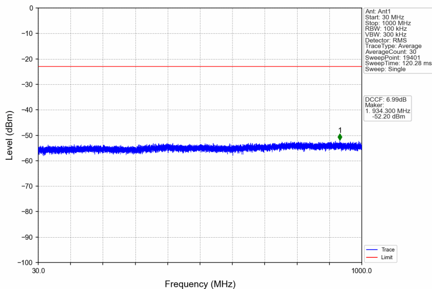
n38_30kHz_SISO_NTNV_30MHz_CP-OFDM QPSK_2585MHz_Edge_1RB_Left
