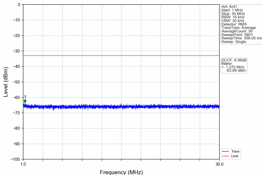
n38_30kHz_SISO_NTNV_30MHz_CP-OFDM QPSK_2585MHz_Edge_1RB_Left
