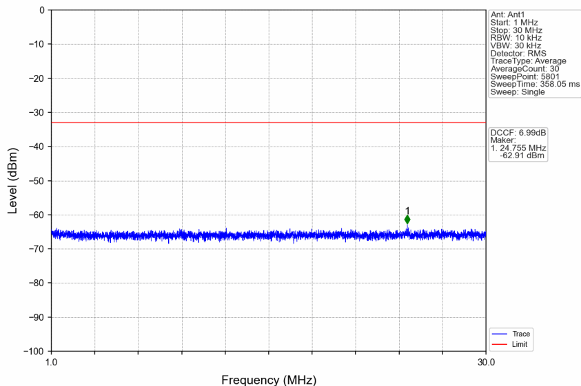
n38_30kHz_SISO_NTNV_20MHz_DFT-s-OFDM QPSK_2595MHz_Edge_1RB_Left
