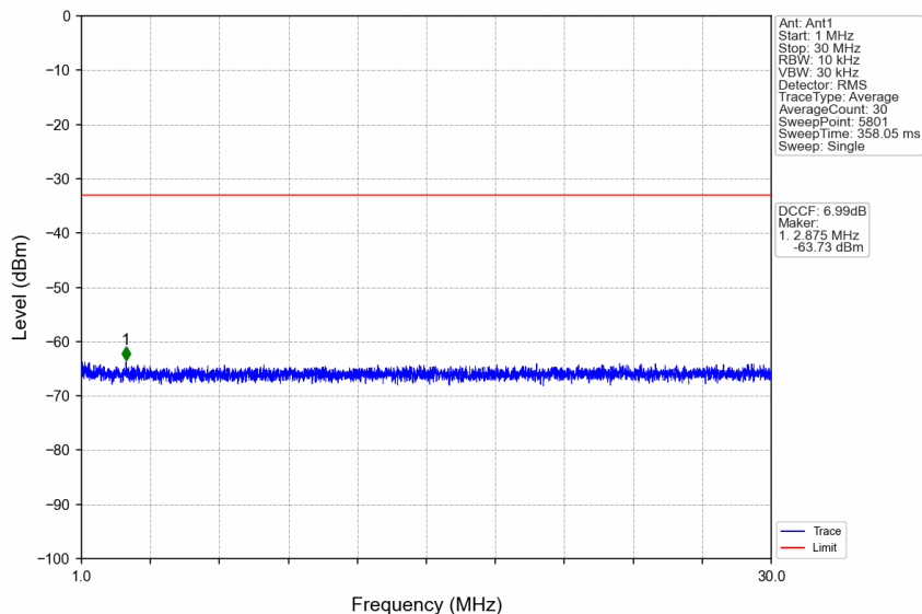
n38_30kHz_SISO_NTNV_20MHz_DFT-s-OFDM QPSK_2580MHz_Edge_1RB_Left
