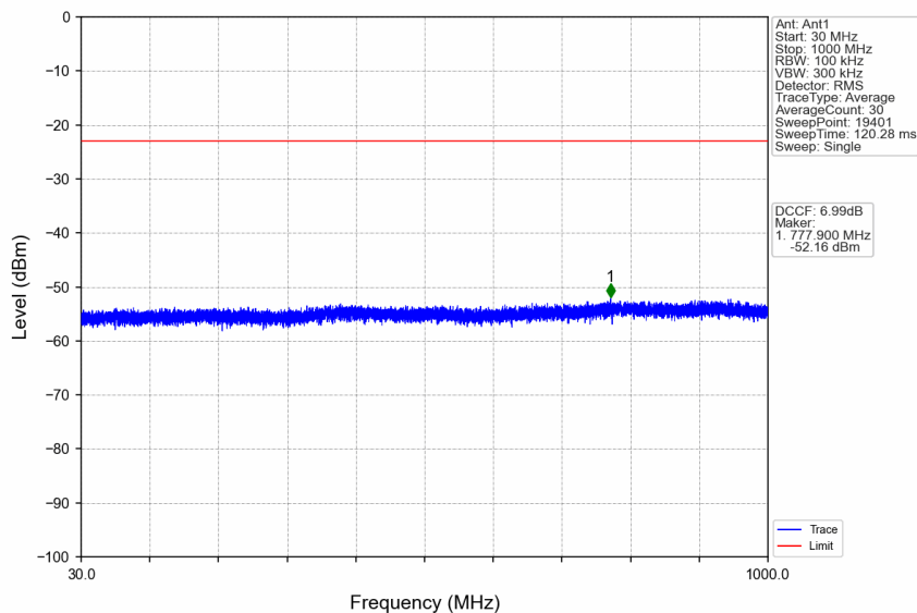
n38_30kHz_SISO_NTNV_20MHz_CP-OFDM QPSK_2595MHz_Edge_1RB_Left
