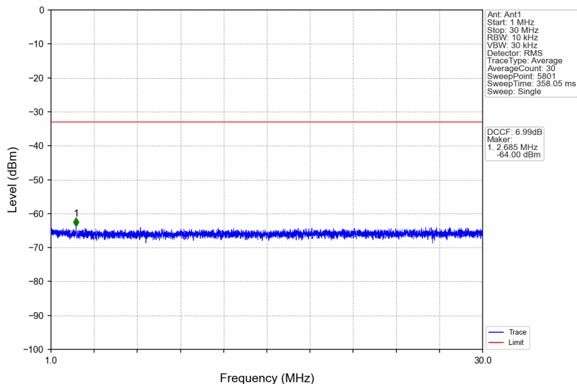
n38_30kHz_SISO_NTNV_20MHz_CP-OFDM QPSK_2580MHz_Edge_1RB_Left
