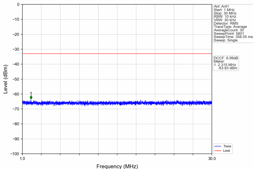
n38_30kHz_SISO_NTNV_20MHz_CP-OFDM QPSK_2595MHz_Edge_1RB_Left
