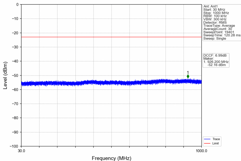
n38_30kHz_SISO_NTNV_20MHz_DFT-s-OFDM QPSK_2580MHz_Edge_1RB_Left
