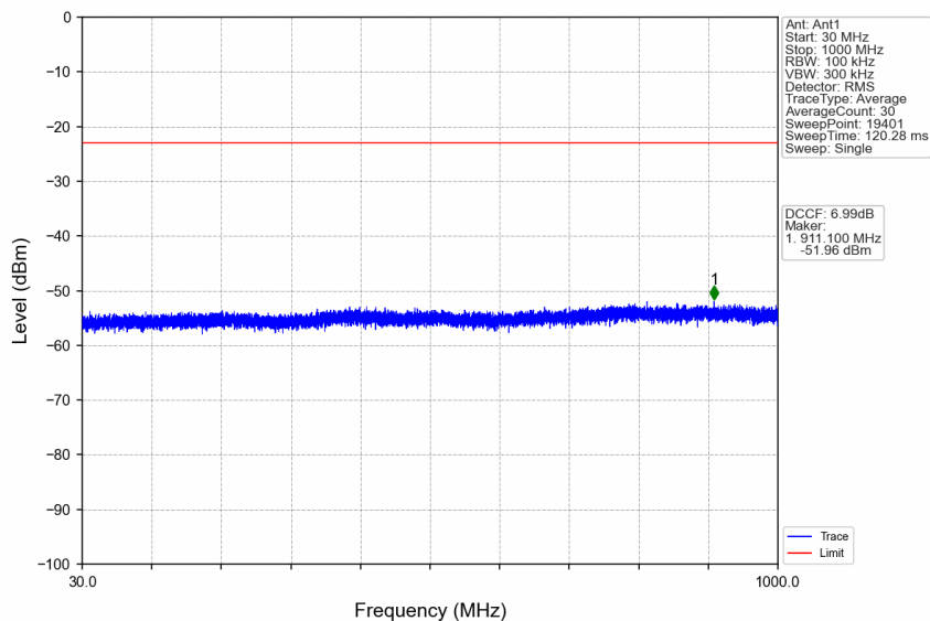
n38_30kHz_SISO_NTNV_10MHz_DFT-s-OFDM QPSK_2595MHz_Edge_1RB_Left
