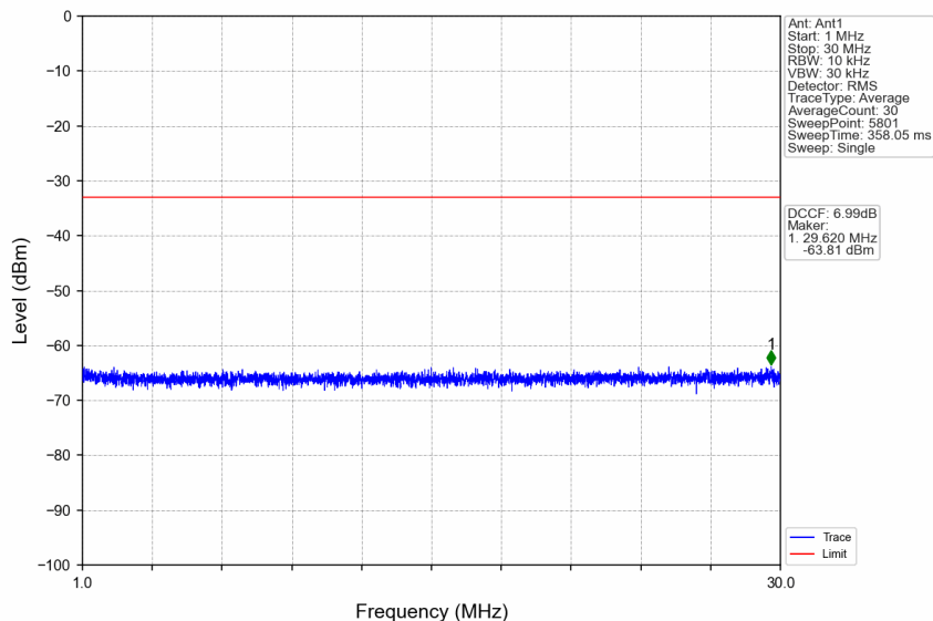
n38_30kHz_SISO_NTNV_10MHz_DFT-s-OFDM QPSK_2595MHz_Edge_1RB_Left
