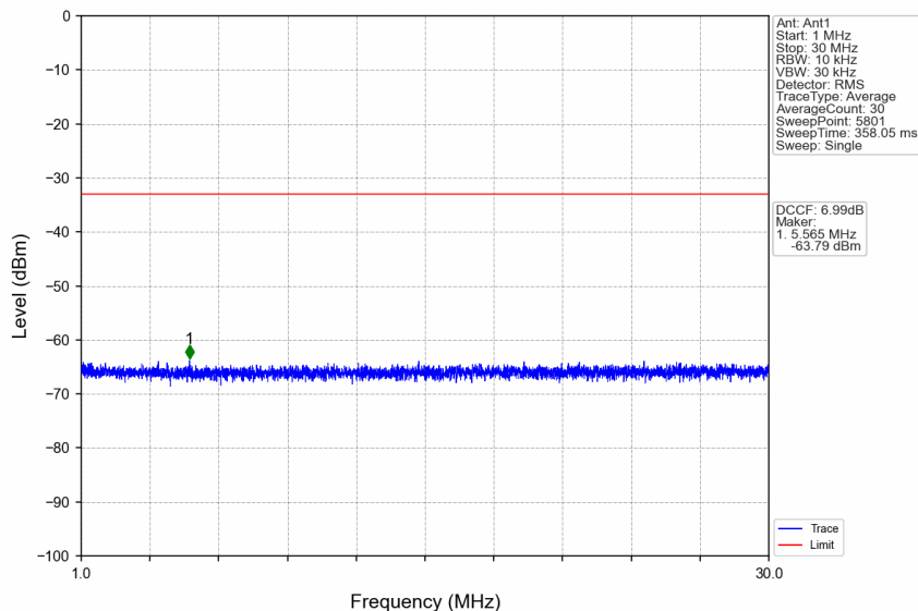
n38_30kHz_SISO_NTNV_10MHz_CP-OFDM QPSK_2595MHz_Edge_1RB_Left
