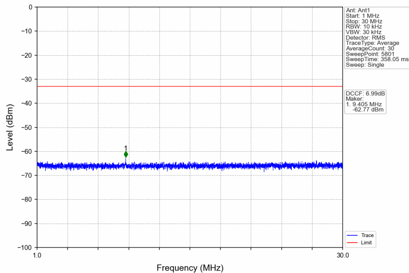
n38_15kHz_SISO_NTNV_40MHz_DFT-s-OFDM QPSK_2590MHz_Edge_1RB_Left
