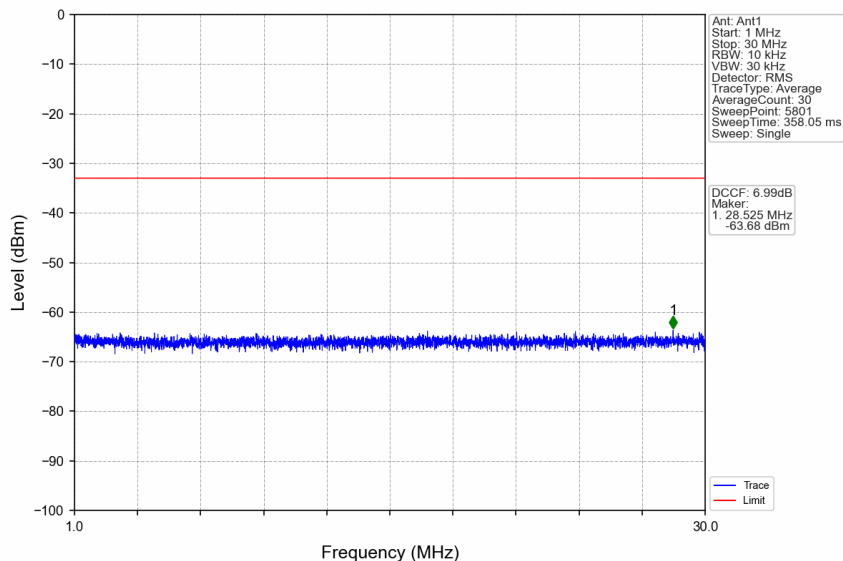
n38_15kHz_SISO_NTNV_40MHz_CP-OFDM QPSK_2590MHz_Edge_1RB_Left
