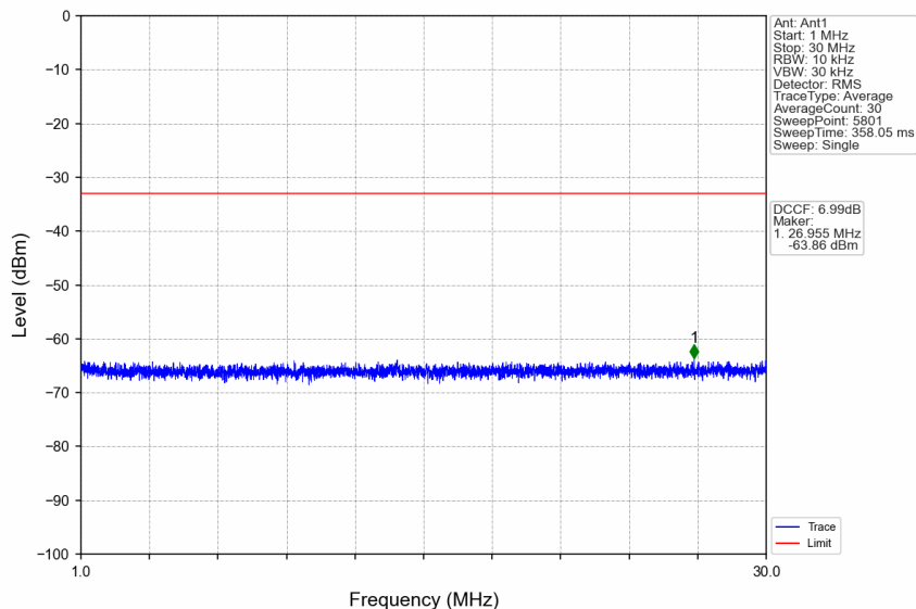
n38_15kHz_SISO_NTNV_40MHz_CP-OFDM QPSK_2595MHz_Edge_1RB_Left
