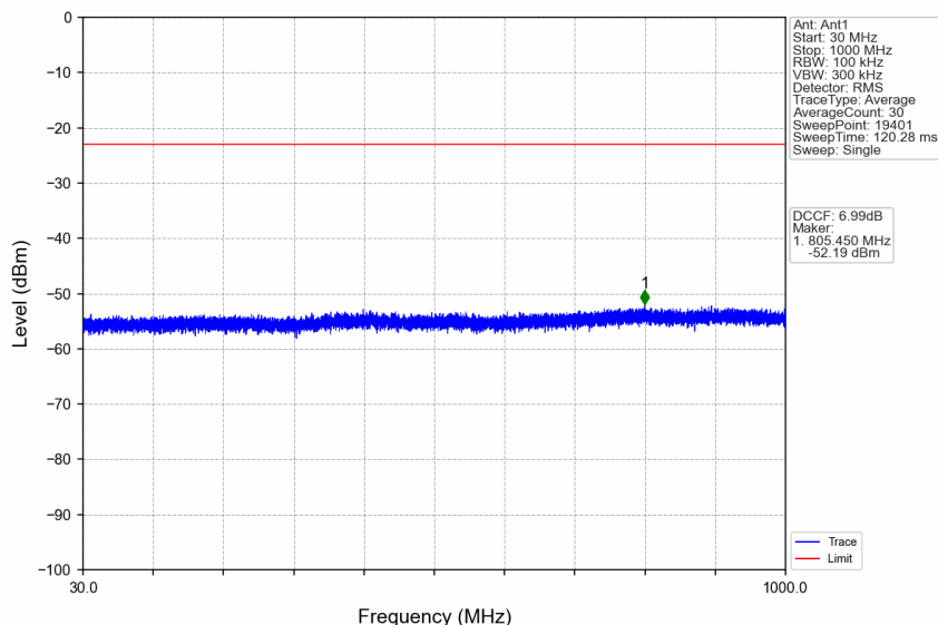
n38_15kHz_SISO_NTNV_20MHz_CP-OFDM QPSK_2595MHz_Edge_1RB_Left
