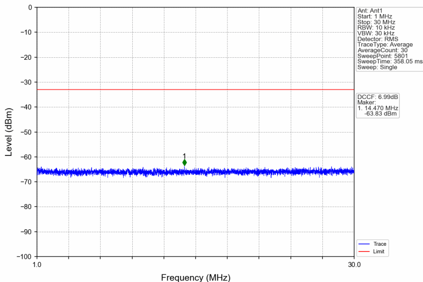
n38_15kHz_SISO_NTNV_20MHz_CP-OFDM QPSK_2580MHz_Edge_1RB_Left
