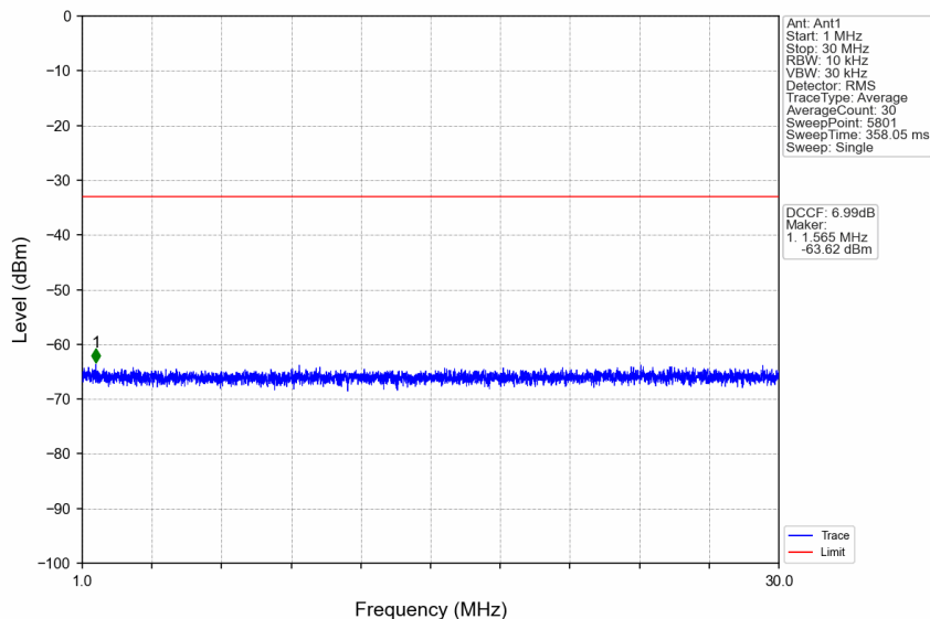
n38_15kHz_SISO_NTNV_20MHz_DFT-s-OFDM QPSK_2595MHz_Edge_1RB_Left
