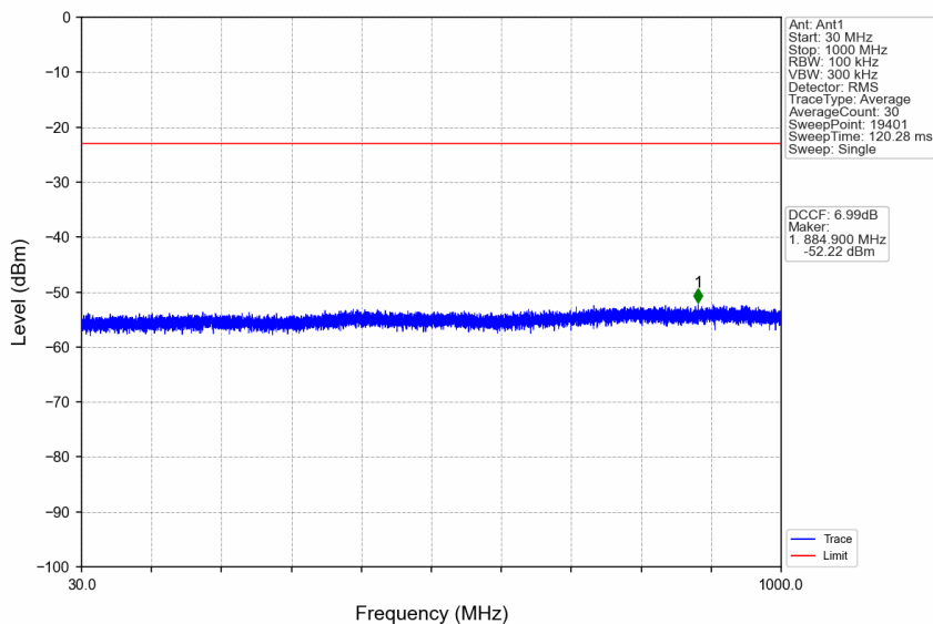
n38_15kHz_SISO_NTNV_20MHz_CP-OFDM QPSK_2580MHz_Edge_1RB_Left
