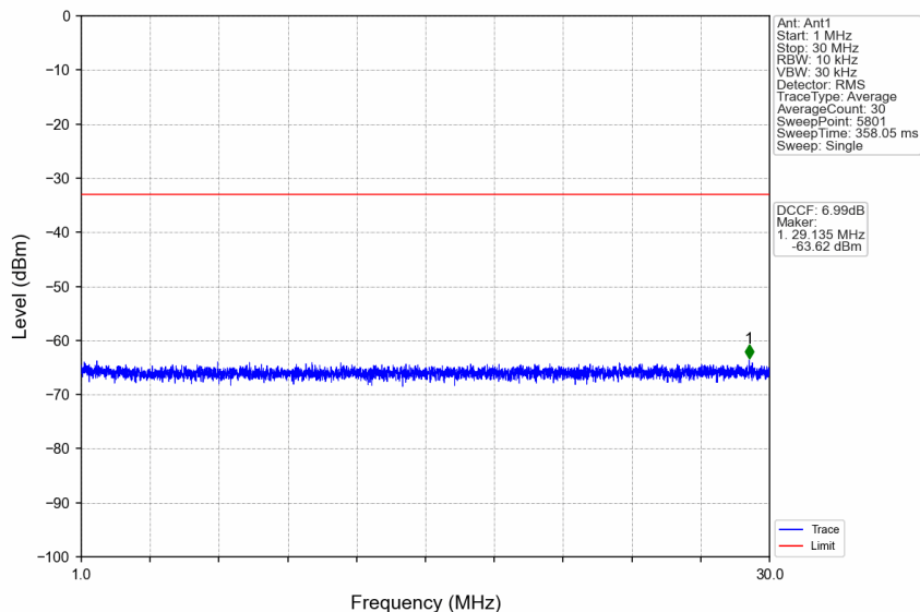
n38_15kHz_SISO_NTNV_10MHz_CP-OFDM QPSK_2595MHz_Edge_1RB_Left
