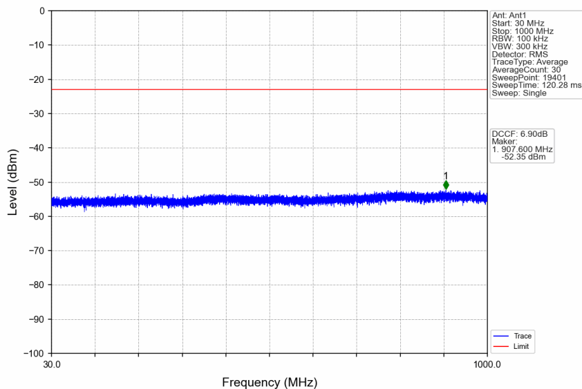
n38_15kHz_SISO_NTNV_5MHz_CP-OFDM QPSK_2595MHz_Edge_1RB_Left
