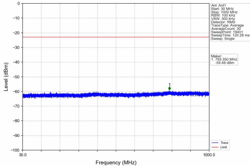
n7_30kHz_SISO_NTNV_20MHz_CP-OFDM QPSK_2510MHz_Edge_1RB_Left
