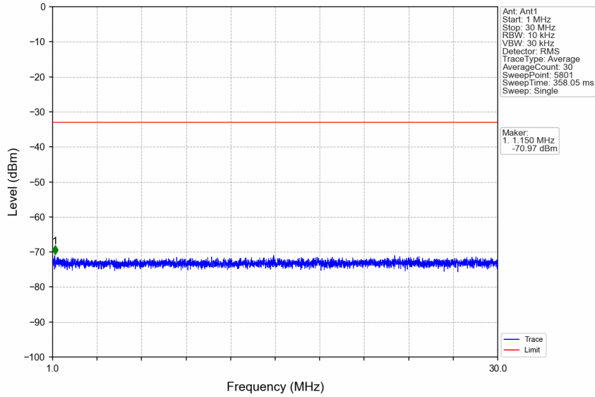
n7_15kHz_SISO_NTNV_20MHz_CP-OFDM QPSK_2535MHz_Edge_1RB_Left
