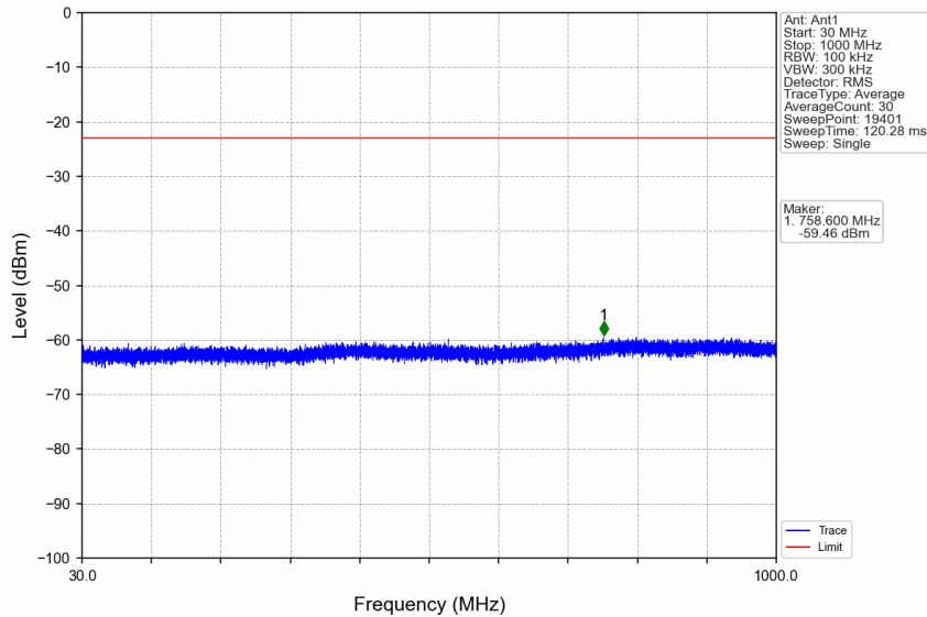
n7_15kHz_SISO_NTNV_20MHz_DFT-s-OFDM QPSK_2510MHz_Edge_1RB_Left
