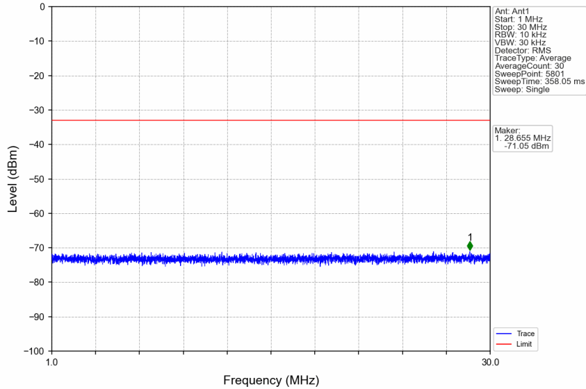
n7_15kHz_SISO_NTNV_20MHz_CP-OFDM QPSK_2510MHz_Edge_1RB_Left
