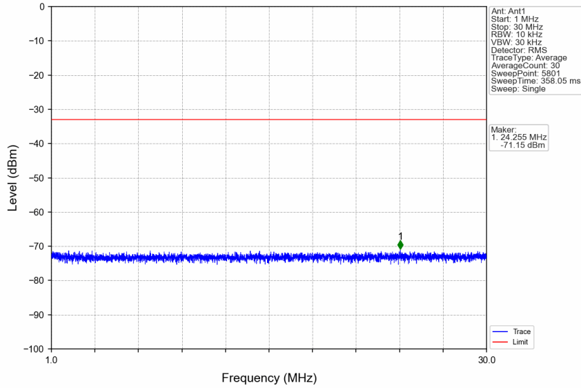
n7_15kHz_SISO_NTNV_20MHz_DFT-s-OFDM QPSK_2510MHz_Edge_1RB_Left
