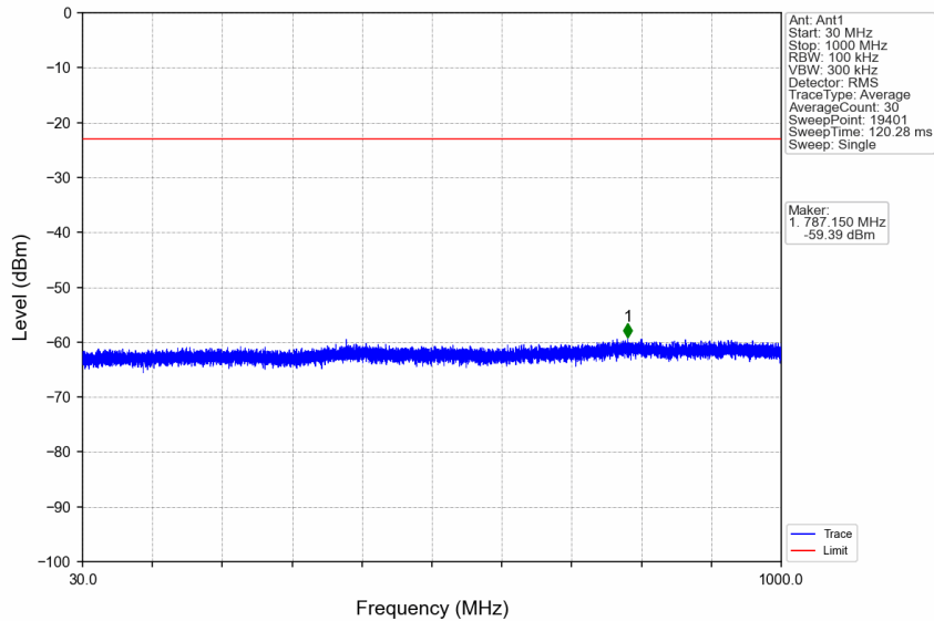
n7_15kHz_SISO_NTNV_20MHz_CP-OFDM QPSK_2535MHz_Edge_1RB_Left
