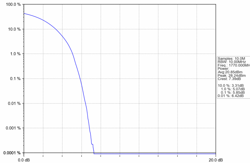
Band66_20MHz_QPSK_HCH_1770MHz_RB_100_0_NTNV
