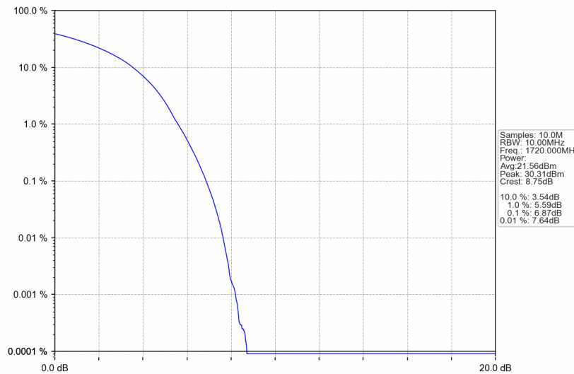
Band66_20MHz_16QAM_LCH_1720MHz_RB_100_0_NTNV
