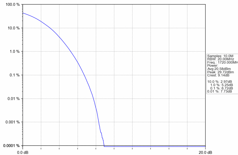
Band66_20MHz_256QAM_LCH_1720MHz_RB_100_0_NTNV
