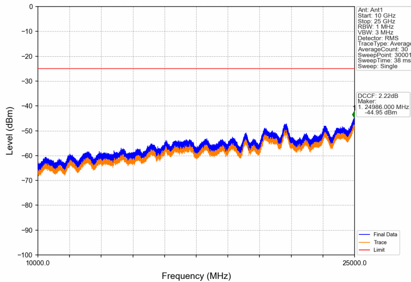
Band41_10MHz_16QAM_LCH_2501MHz_RB_1_0_NTNV
