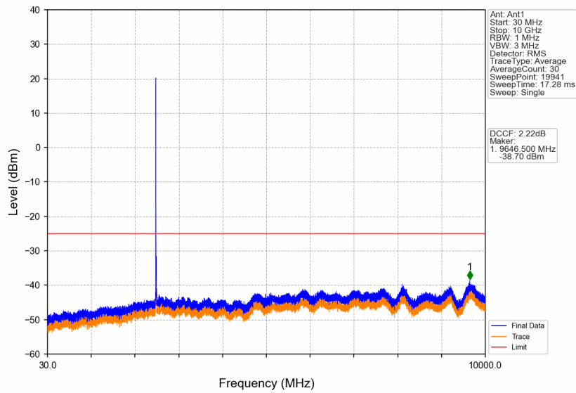
Band41_10MHz_16QAM_LCH_2501MHz_RB_1_0_NTNV
