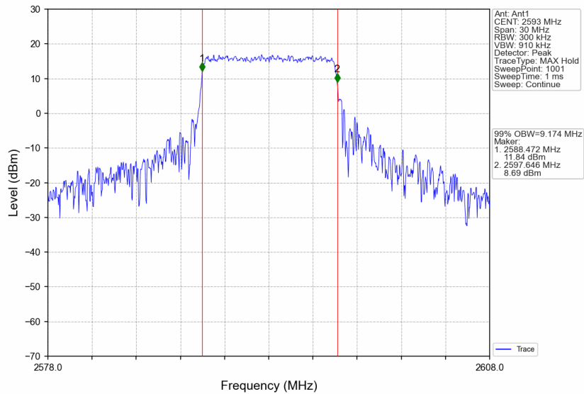
Band41_10MHz_QPSK_MCH_2593MHz_RB_50_0_NTNV
