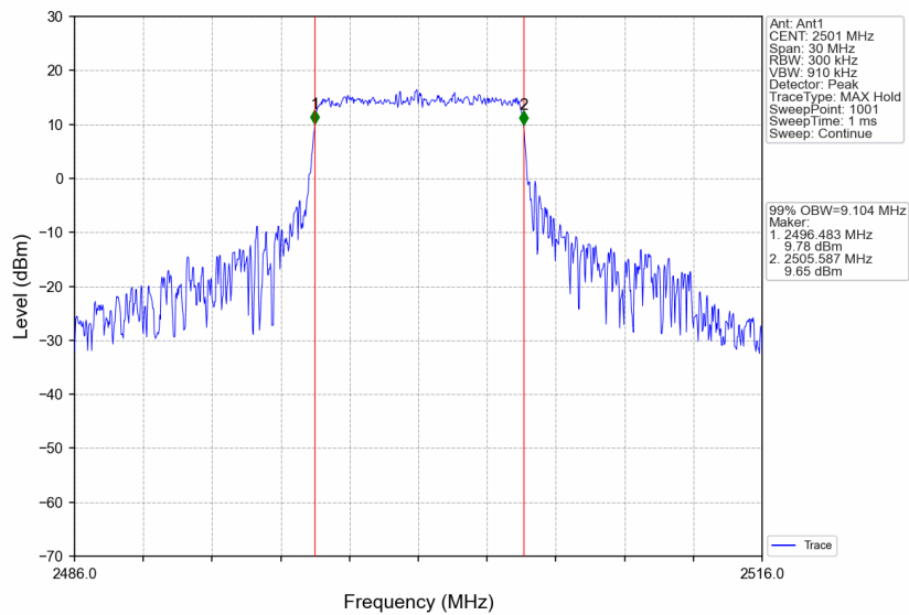
Band41_10MHz_256QAM_LCH_2501MHz_RB_50_0_NTNV
