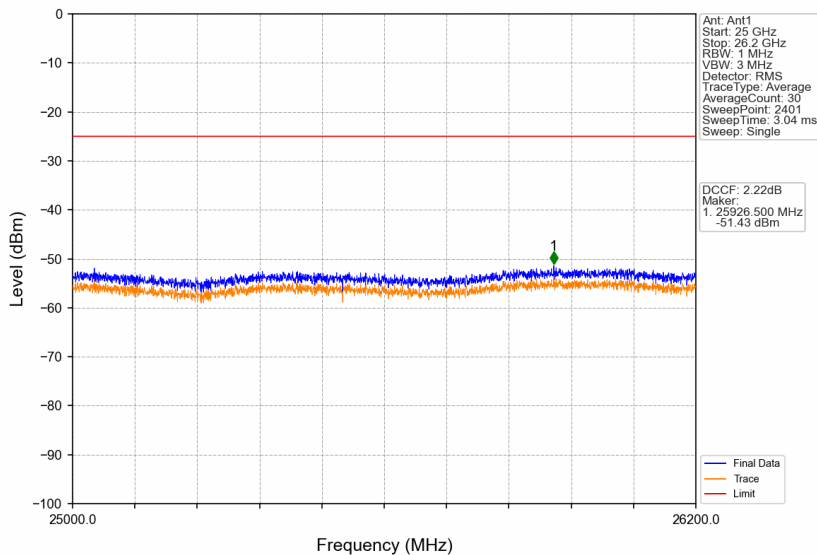
Band38_20MHz_256QAM_HCH_2610MHz_RB_1_0_NTNV
