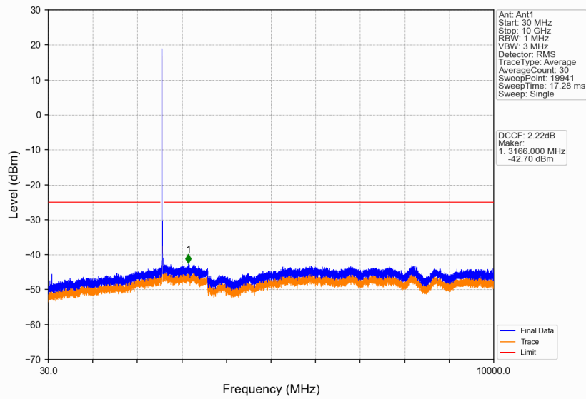
Band38_20MHz_256QAM_LCH_2580MHz_RB_1_0_NTNV
