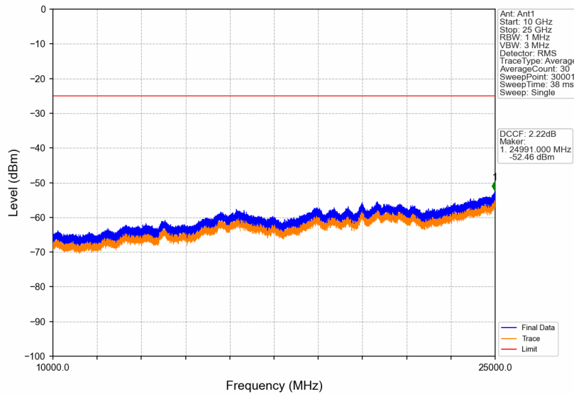
Band38_20MHz_256QAM_LCH_2580MHz_RB_1_0_NTNV
