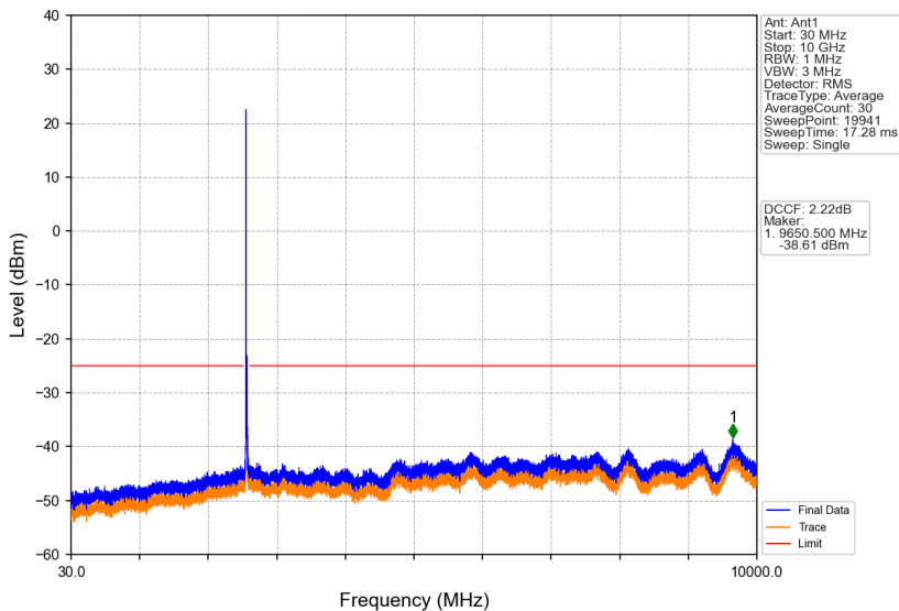
Band38_20MHz_16QAM_LCH_2580MHz_RB_1_0_NTNV
