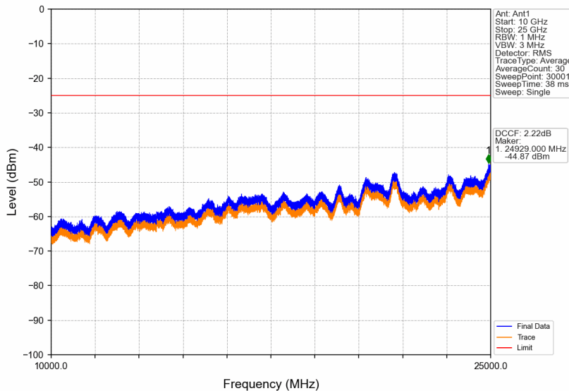
Band38_20MHz_16QAM_LCH_2580MHz_RB_1_0_NTNV
