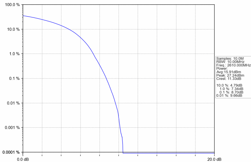
Band38_20MHz_16QAM_HCH_2610MHz_RB_100_0_NTNV
