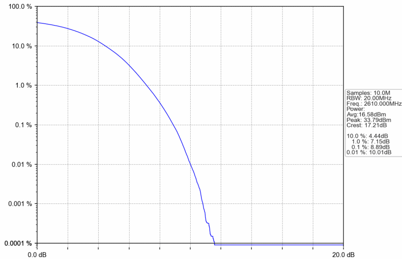
Band38_20MHz_256QAM_HCH_2610MHz_RB_100_0_NTNV
