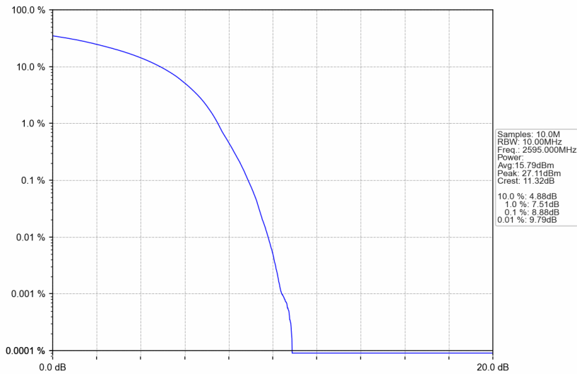
Band38_20MHz_16QAM_MCH_2595MHz_RB_100_0_NTNV
