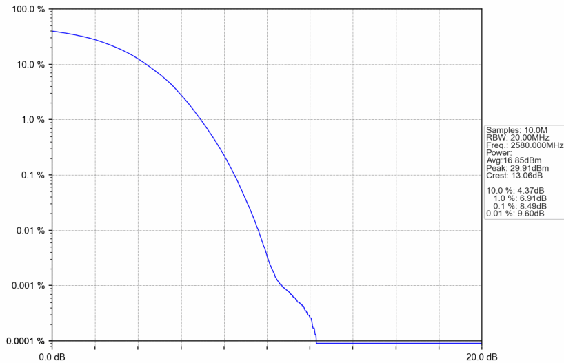
Band38_20MHz_256QAM_LCH_2580MHz_RB_100_0_NTNV
