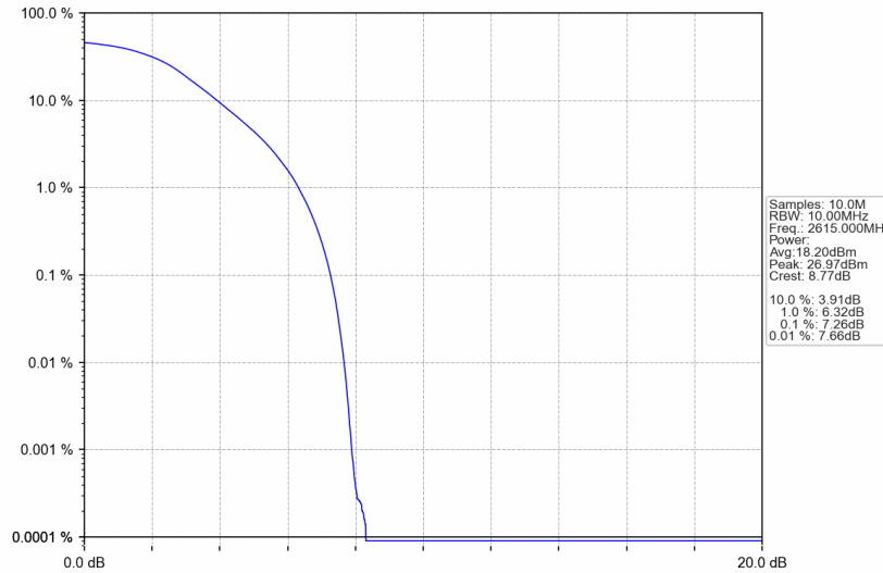
Band38_10MHz_QPSK_HCH_2615MHz_RB_50_0_NTNV
