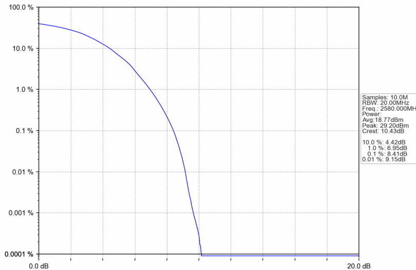
Band38_20MHz_64QAM_LCH_2580MHz_RB_100_0_NTNV
