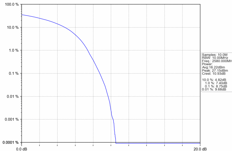
Band38_20MHz_16QAM_LCH_2580MHz_RB_100_0_NTNV
