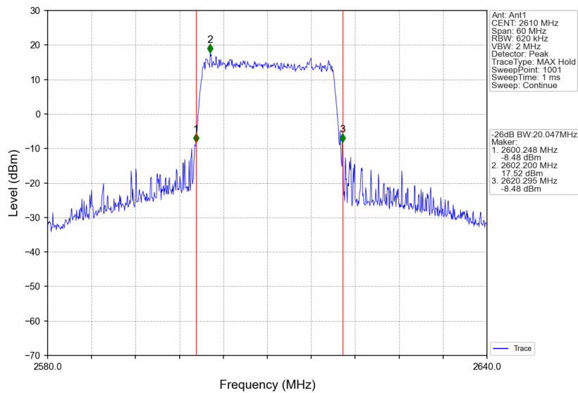
Band38_20MHz_256QAM_HCH_2610MHz_RB_100_0_NTNV
