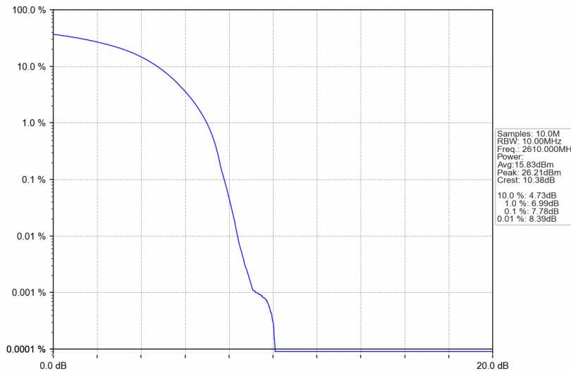
Band38_20MHz_QPSK_HCH_2610MHz_RB_100_0_NTNV
