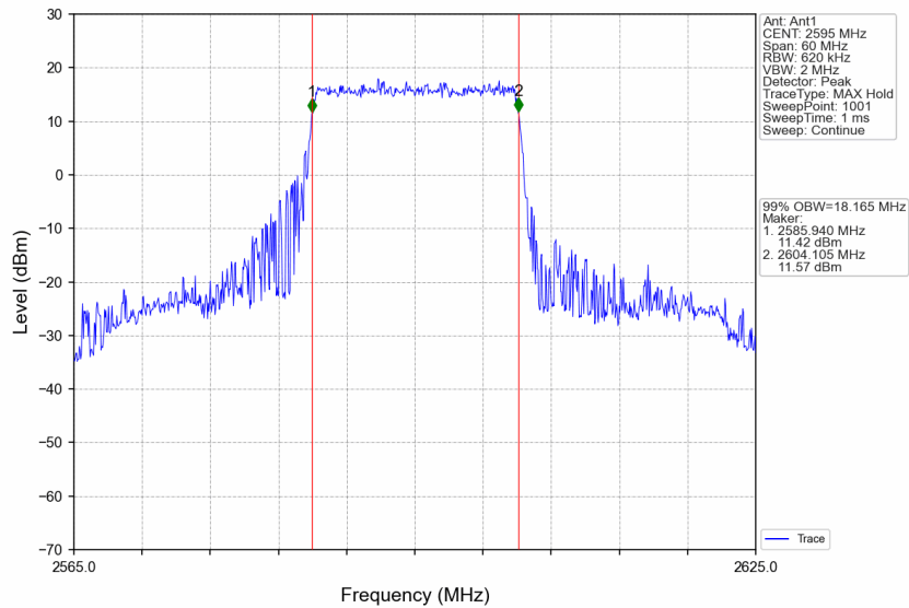
Band38_20MHz_QPSK_MCH_2595MHz_RB_100_0_NTNV
