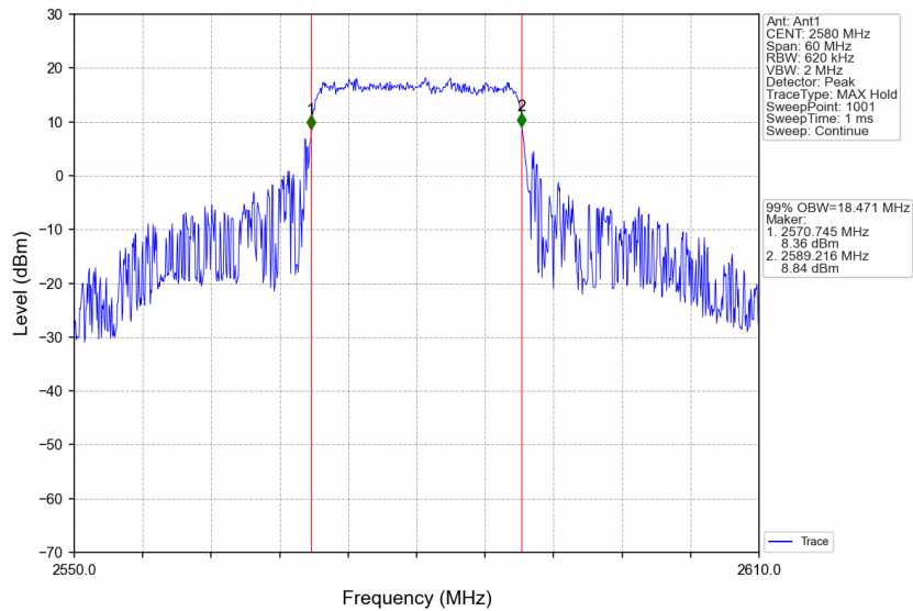
Band38_20MHz_16QAM_LCH_2580MHz_RB_100_0_NTNV
