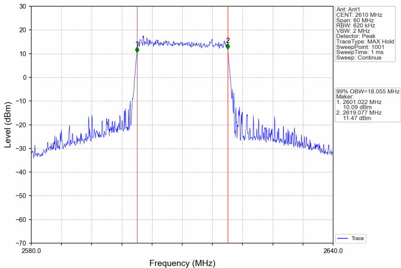
Band38_20MHz_256QAM_HCH_2610MHz_RB_100_0_NTNV
