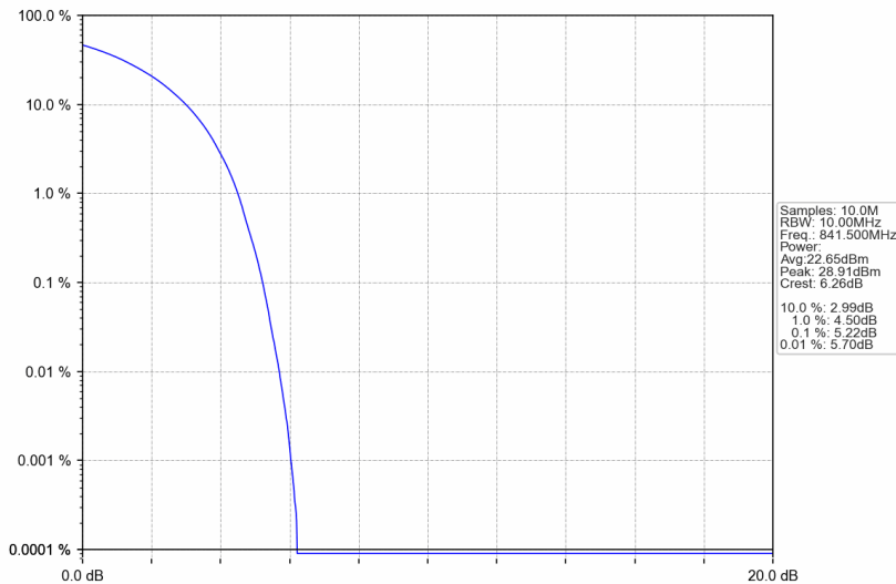
Band26c_15MHz_QPSK_HCH_841.5MHz_RB_75_0_NTNV
