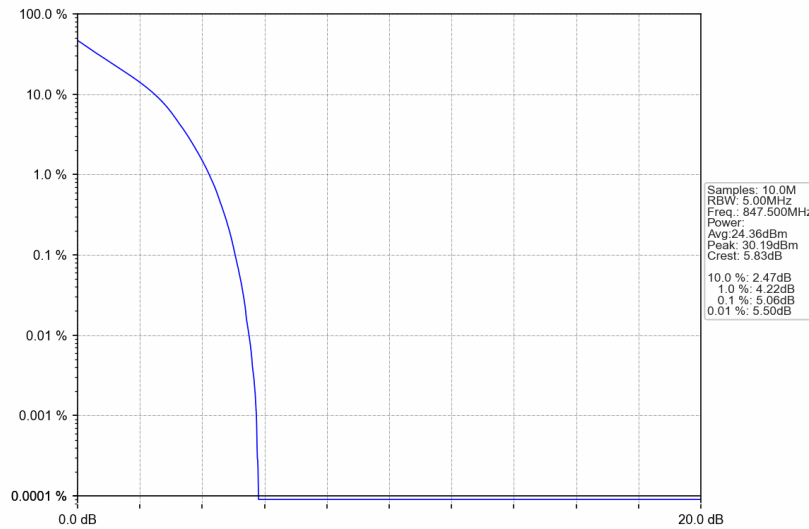
Band26b_3MHz_QPSK_HCH_847.5MHz_RB_15_0_NTNV
