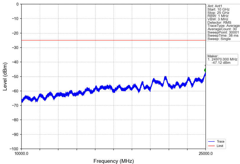
Band7_20MHz_16QAM_HCH_2560MHz_RB_1_0_NTNV
