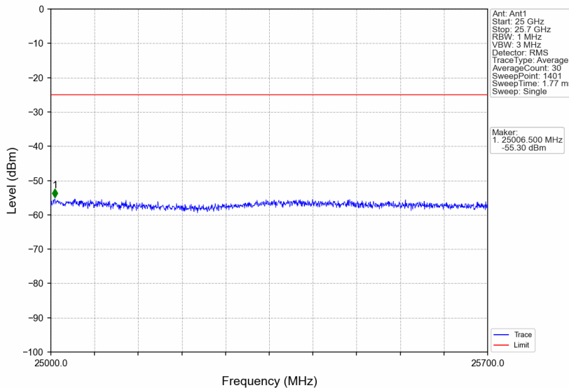
Band7_20MHz_64QAM_MCH_2535MHz_RB_1_0_NTNV
