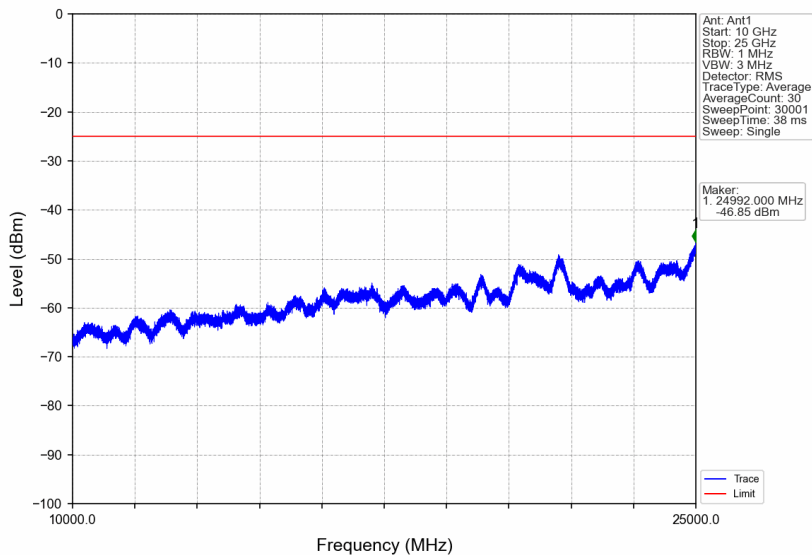
Band7_20MHz_QPSK_LCH_2510MHz_RB_1_0_NTNV
