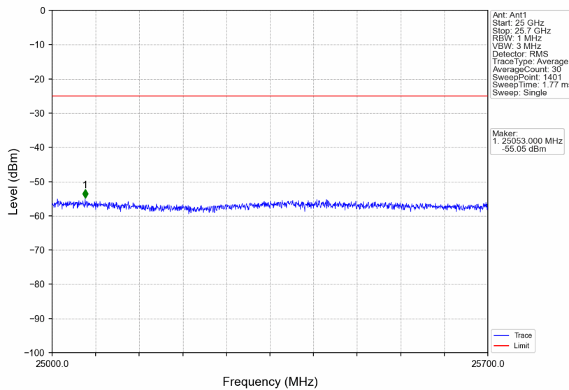
Band7_20MHz_256QAM_HCH_2560MHz_RB_1_0_NTNV
