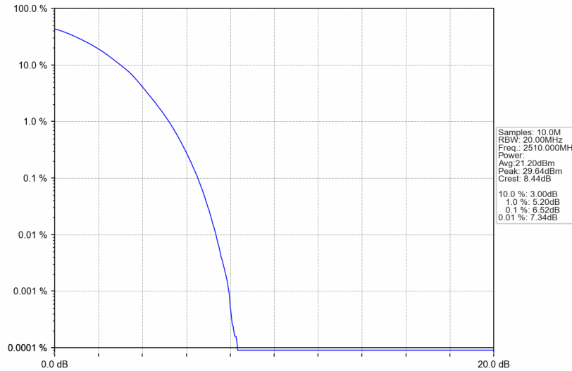
Band7_20MHz_64QAM_LCH_2510MHz_RB_100_0_NTNV
