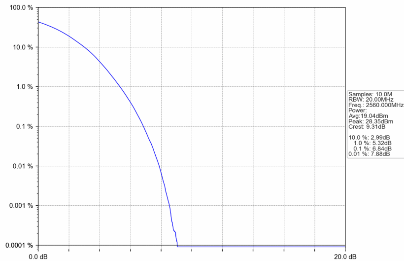
Band7_20MHz_256QAM_HCH_2560MHz_RB_100_0_NTNV
