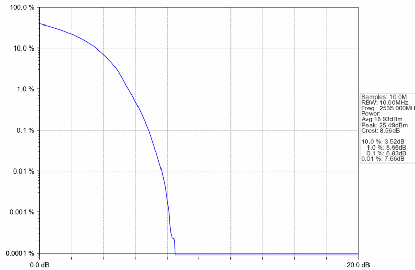
Band7_20MHz_16QAM_MCH_2535MHz_RB_100_0_NTNV
