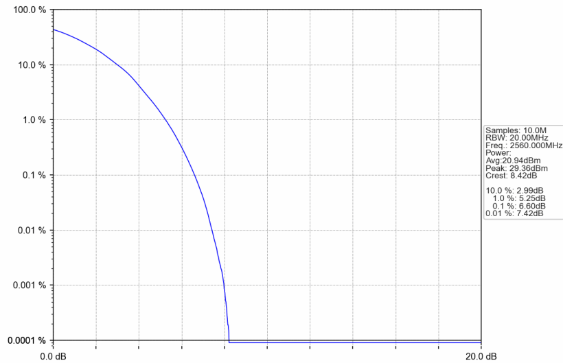
Band7_20MHz_64QAM_HCH_2560MHz_RB_100_0_NTNV
