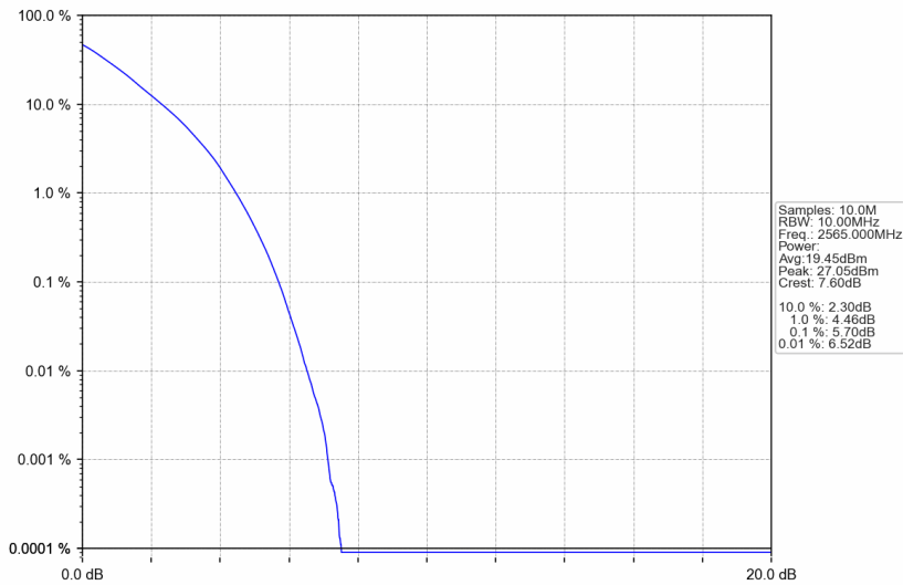
Band7_10MHz_QPSK_HCH_2565MHz_RB_50_0_NTNV
