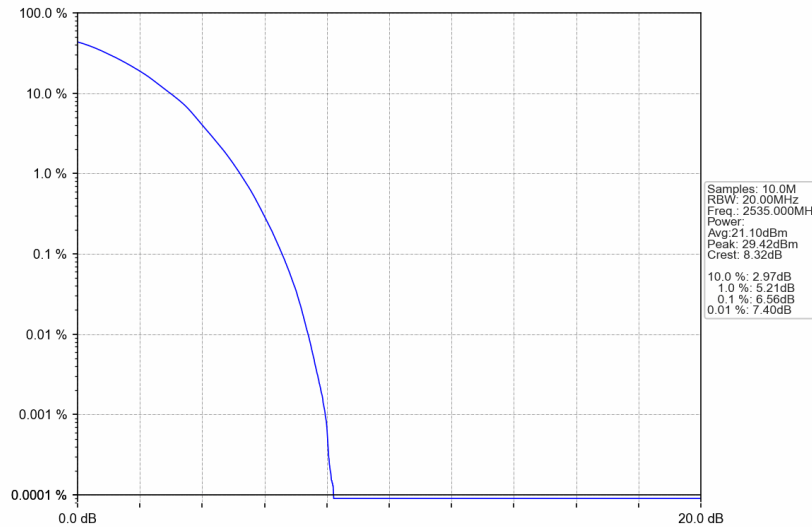
Band7_20MHz_64QAM_MCH_2535MHz_RB_100_0_NTNV
