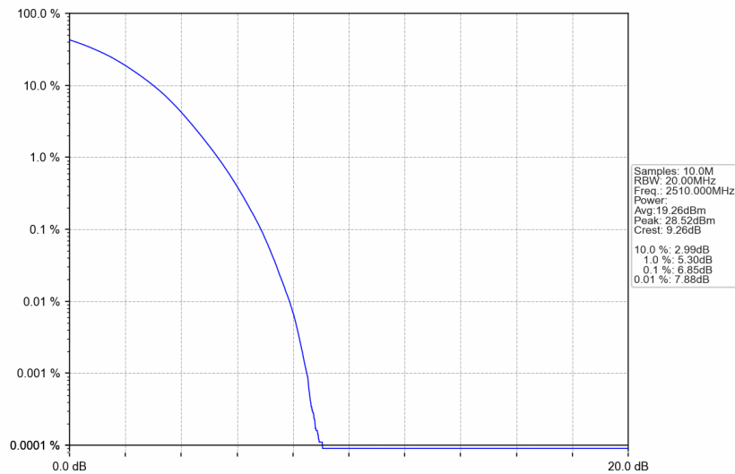
Band7_20MHz_256QAM_LCH_2510MHz_RB_100_0_NTNV
