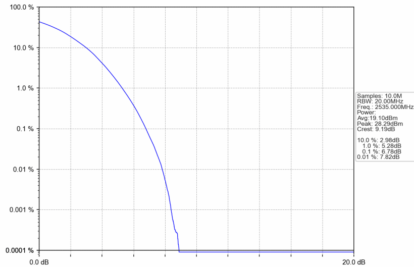
Band7_20MHz_256QAM_MCH_2535MHz_RB_100_0_NTNV
