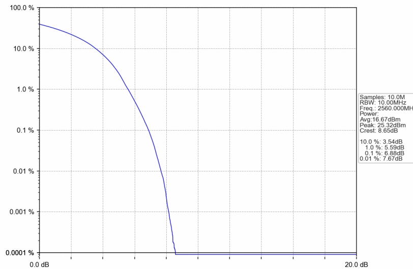
Band7_20MHz_16QAM_HCH_2560MHz_RB_100_0_NTNV
