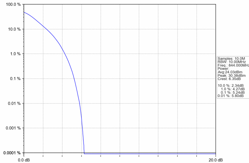
Band5_10MHz_QPSK_HCH_844MHz_RB_50_0_NTNV
