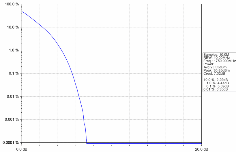
Band4_10MHz_QPSK_HCH_1750MHz_RB_50_0_NTNV
