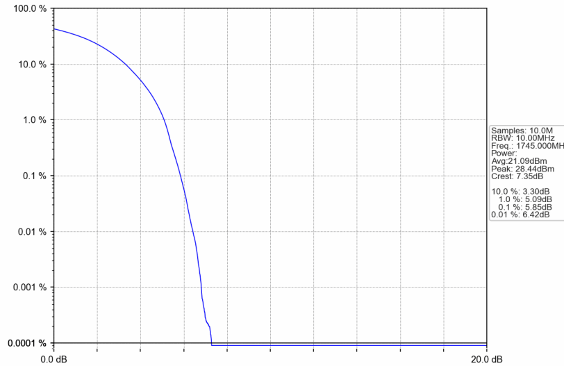
Band4_20MHz_QPSK_HCH_1745MHz_RB_100_0_NTNV
