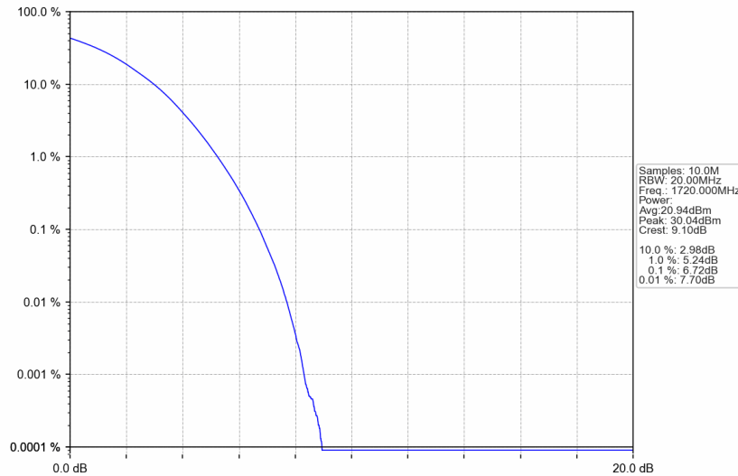
Band4_20MHz_256QAM_LCH_1720MHz_RB_100_0_NTNV
