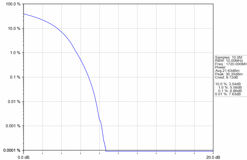
Band4_20MHz_16QAM_LCH_1720MHz_RB_100_0_NTNV
