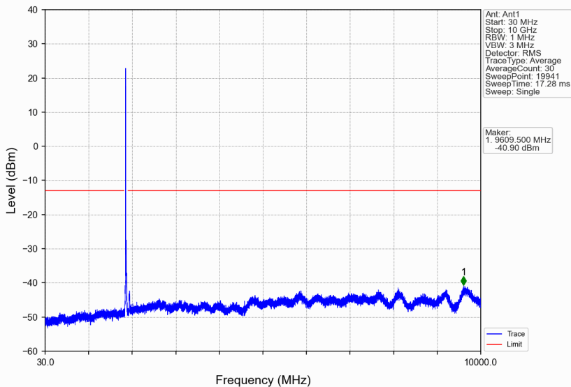
Band2_20MHz_16QAM_MCH_1880MHz_RB_1_0_NTNV
