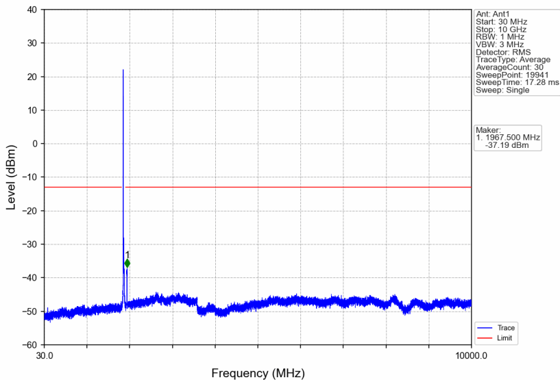
Band2_20MHz_64QAM_MCH_1880MHz_RB_1_0_NTNV
