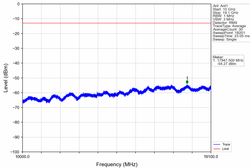
Band2_15MHz_QPSK_HCH_1902.5MHz_RB_1_0_NTNV
