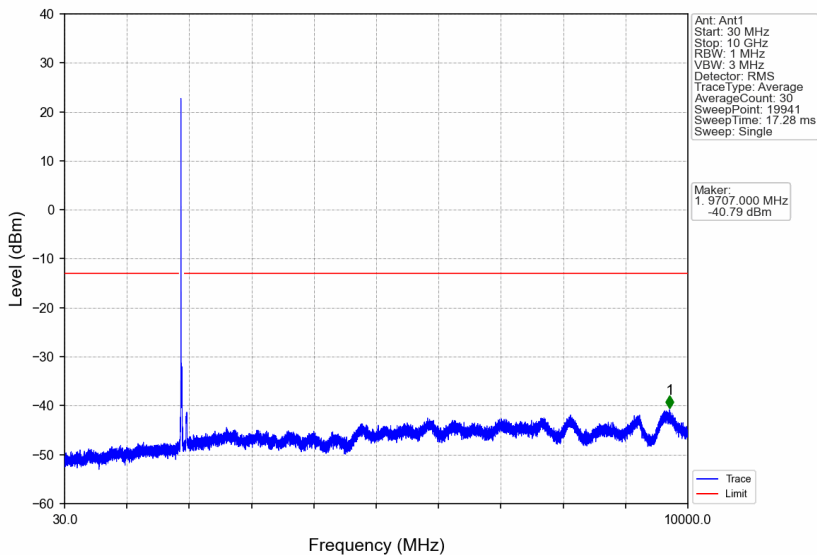
Band2_20MHz_QPSK_HCH_1900MHz_RB_1_0_NTNV
