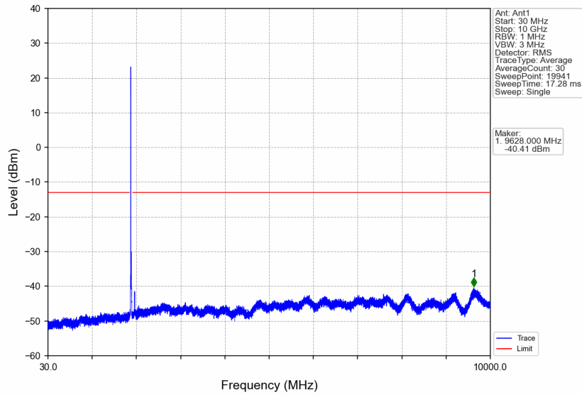
Band2_15MHz_QPSK_HCH_1902.5MHz_RB_1_0_NTNV
