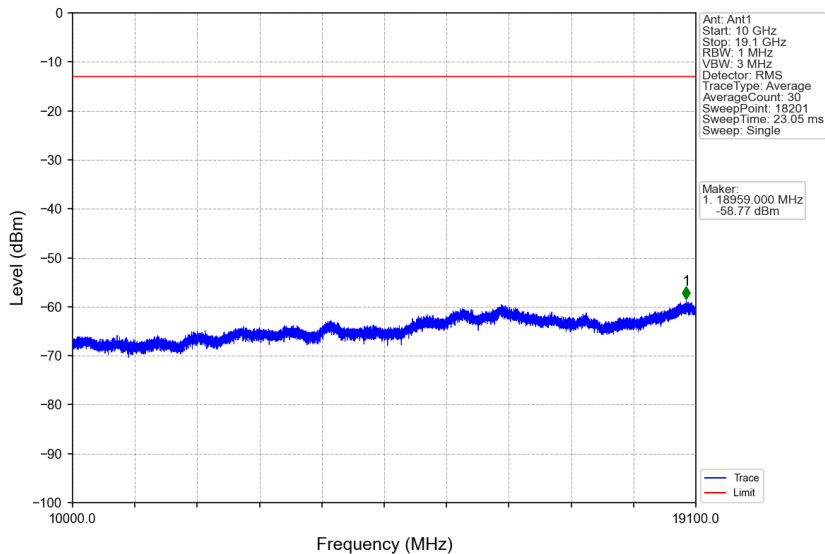
Band2_3MHz_256QAM_HCH_1908.5MHz_RB_1_0_NTNV
