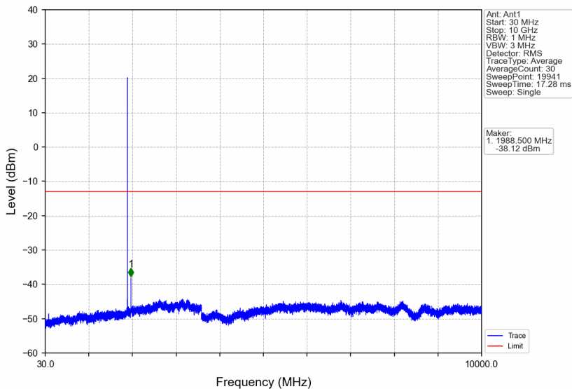
Band2_3MHz_256QAM_HCH_1908.5MHz_RB_1_0_NTNV
