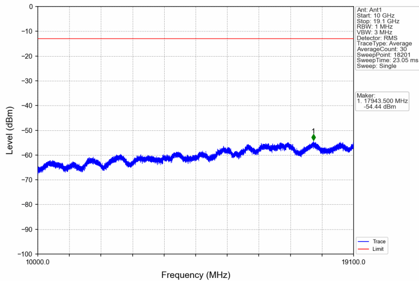
Band2_10MHz_QPSK_HCH_1905MHz_RB_1_0_NTNV
