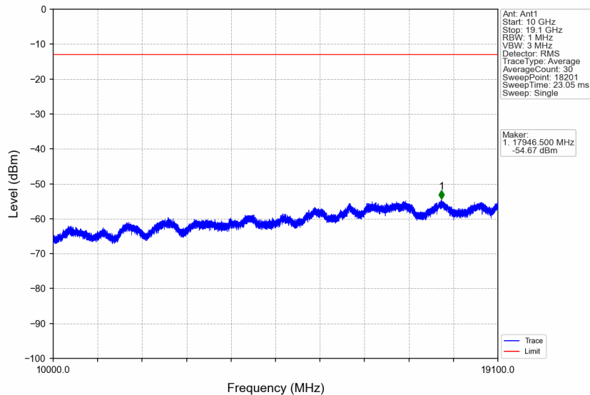
Band2_5MHz_QPSK_MCH_1880MHz_RB_1_0_NTNV
