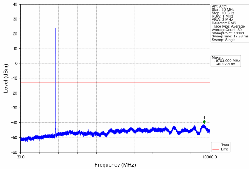
Band2_10MHz_QPSK_MCH_1880MHz_RB_1_0_NTNV
