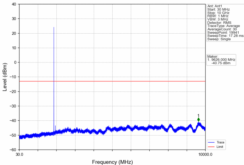
Band2_3MHz_16QAM_MCH_1880MHz_RB_1_0_NTNV
