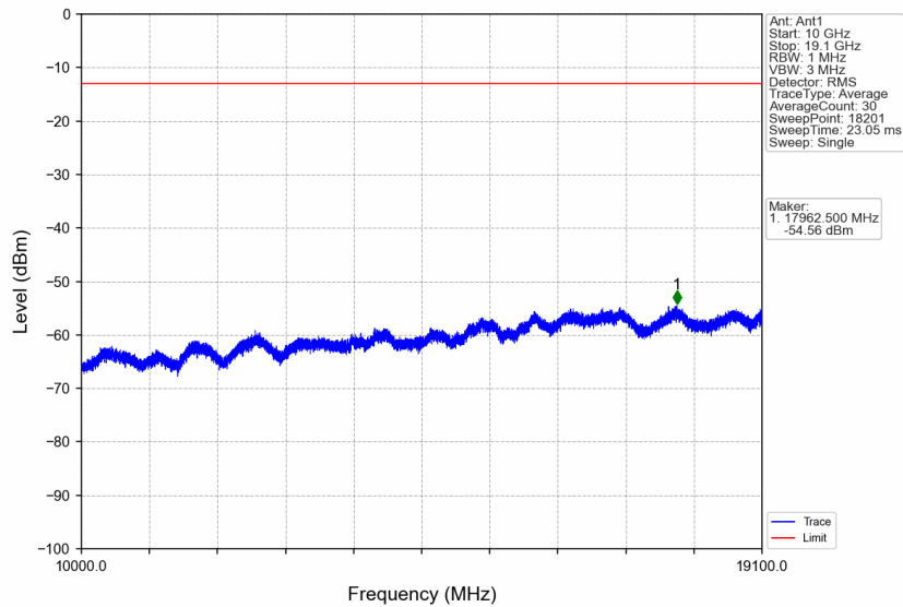
Band2_10MHz_QPSK_MCH_1880MHz_RB_1_0_NTNV
