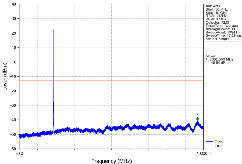
Band2_10MHz_16QAM_MCH_1880MHz_RB_1_0_NTNV
