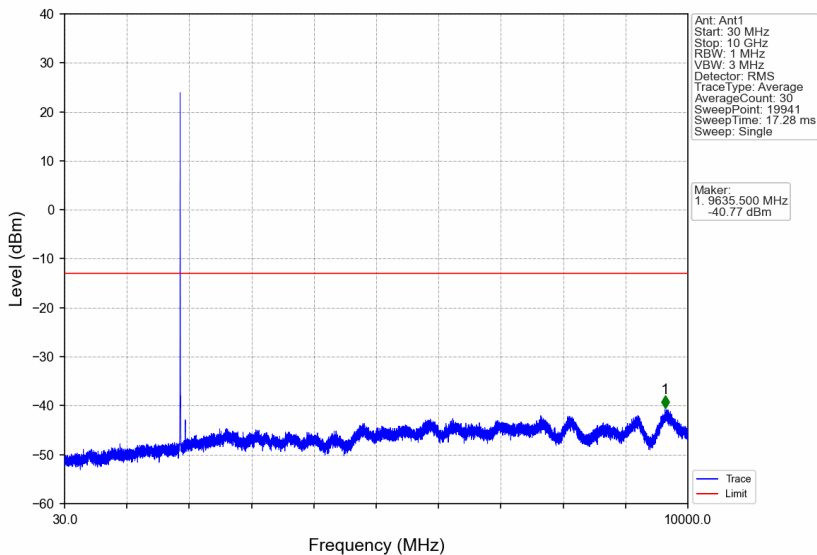
Band2_5MHz_QPSK_MCH_1880MHz_RB_1_0_NTNV
