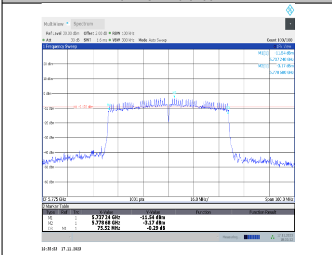
11ac80SISO-Ant6-5775-PASS
