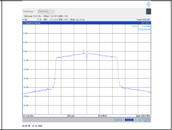
11ac80SISO-Ant6-5530-PASS
