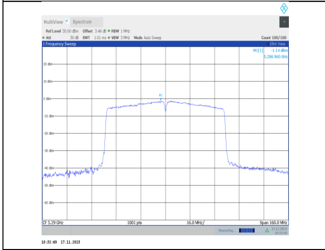
11ac80SISO-Ant6-5290-PASS
