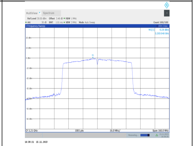
11ac80SISO-Ant6-5210-PASS
