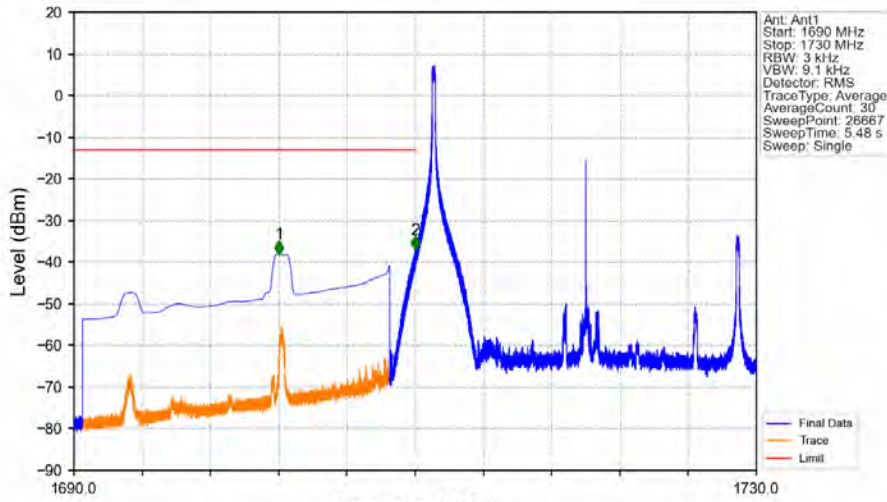
Band66_20MHz_16QAM_LCH_1720MHz_RB_1_0_NTNV
