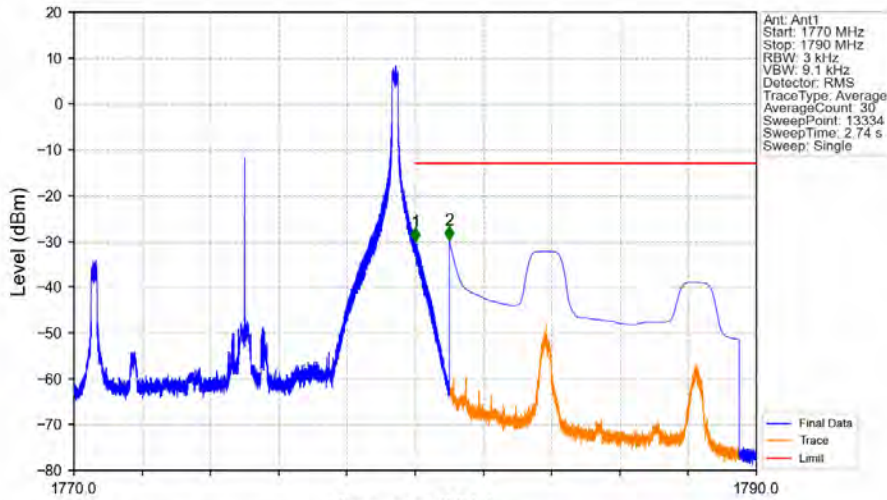
Band66_10MHz_QPSK_HCH_1775MHz_RB_1_49_NTNV
