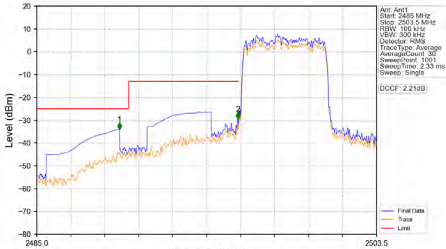
Band41_5MHz_QPSK_LCH_2498.5MHz_RB_25_0_NTNV
