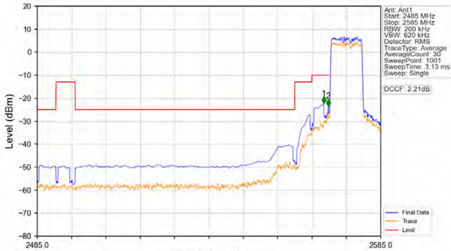
Band38_10MHz_QPSK_LCH_2575MHz_RB_50_0_NTNV
