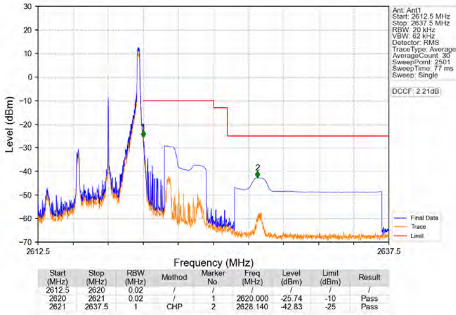
Band38_5MHz_QPSK_HCH_2617.5MHz_RB_1_24_NTNV
