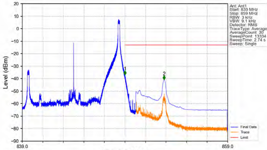
Band26b_10MHz_QPSK_HCH_844MHz_RB_1_49_NTNV
