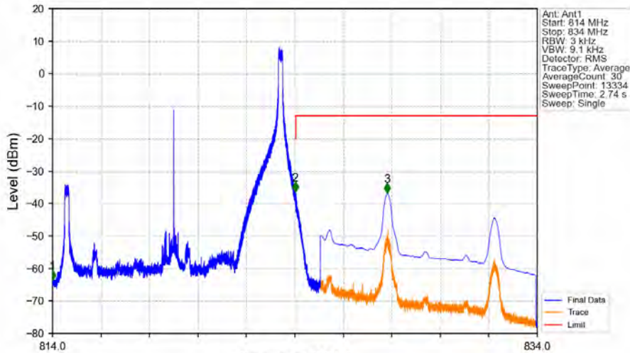
Band26a_10MHz_QPSK_MCH_819MHz_RB_1_49_NTNV
