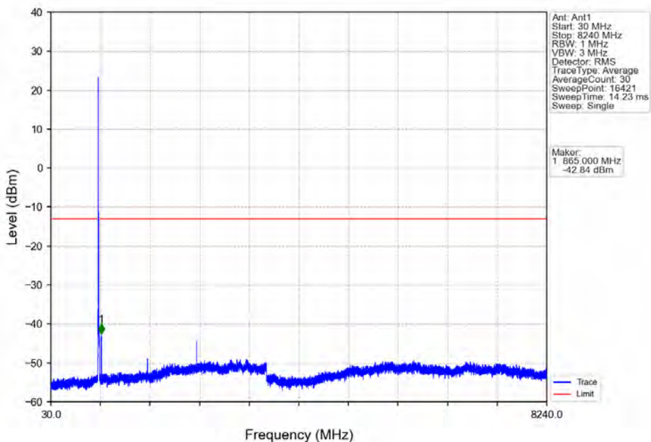
Band26a_10MHz_QPSK_HCH_819MHz_RB_1_0_NTNV
