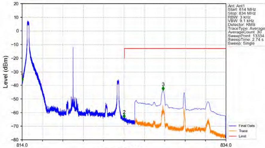
Band26a_10MHz_QPSK_MCH_819MHz_RB_1_0_NTNV
