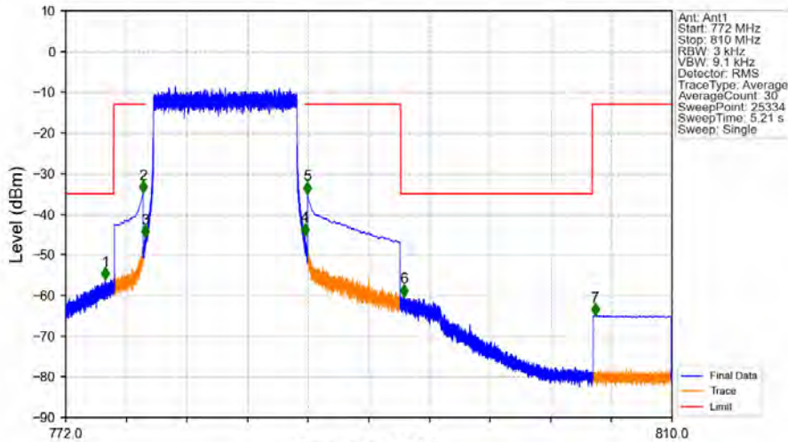
Band13 10MHz QPSK HCH 782MHz RB 50_0 NTV
