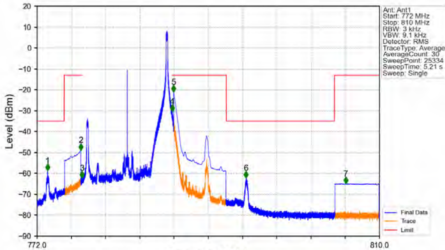
Band13 10MHz QPSK HCH 782MHz RB 1 49 NTV
