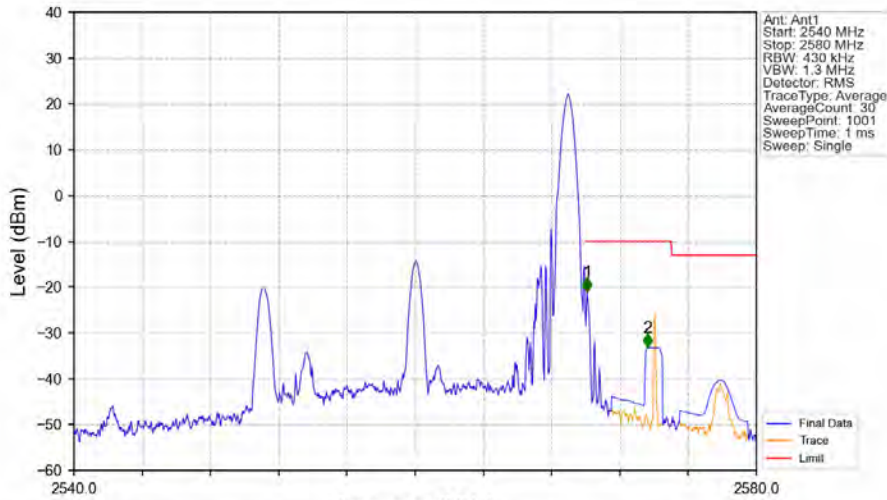
Band7_20MHz_16QAM_HCH_2560MHz_RB_1_99_NTNV
