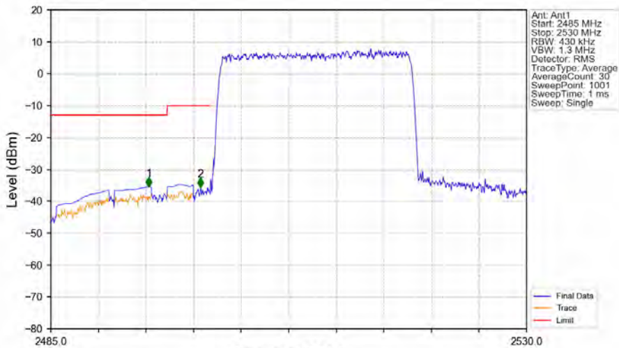
Band7_20MHz_QPSK_LCH_2510MHz_RB_100_0_NTNV
