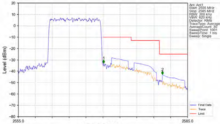
Band7_10MHz_QPSK_HCH_2565MHz_RB_50_0_NTNV
