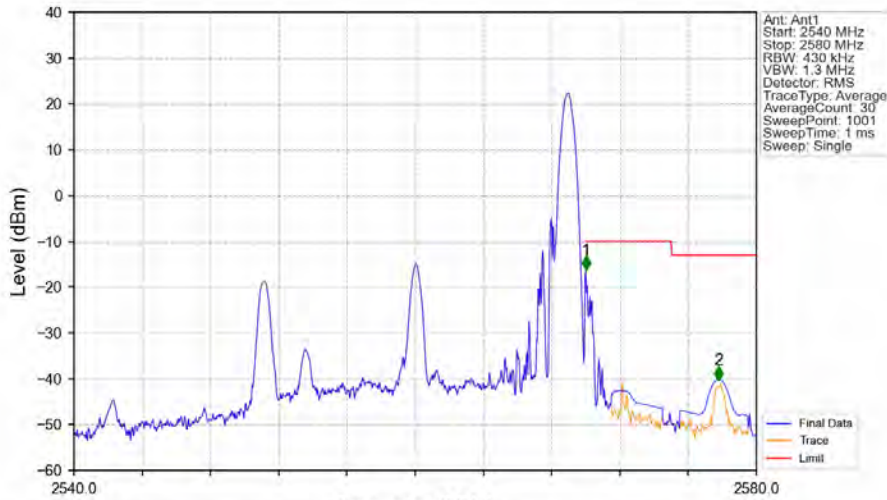
Band7 20MHz QPSK HCH 2560MHz RB 1 99 NTV
