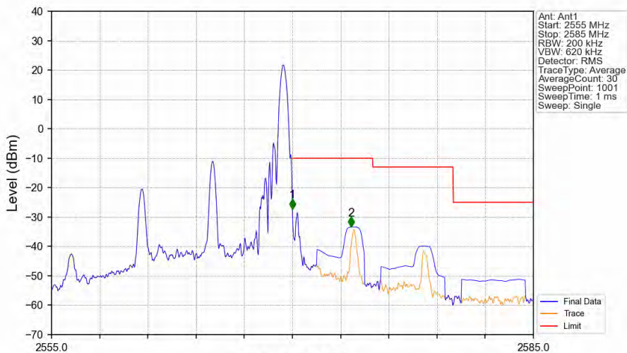
Band7_10MHz_QPSK_HCH_2565MHz_RB_1_49_NTNV
