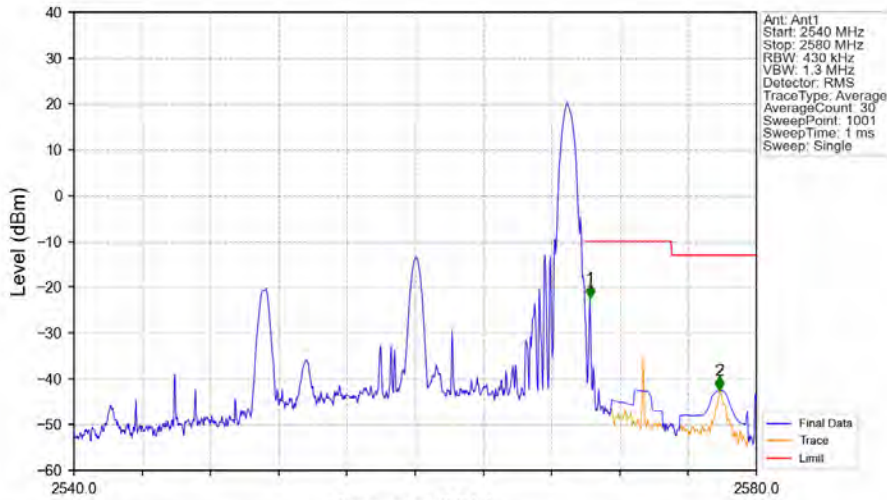
Band7_20MHz_64QAM_HCH_2560MHz_RB_1_99_NTNV
