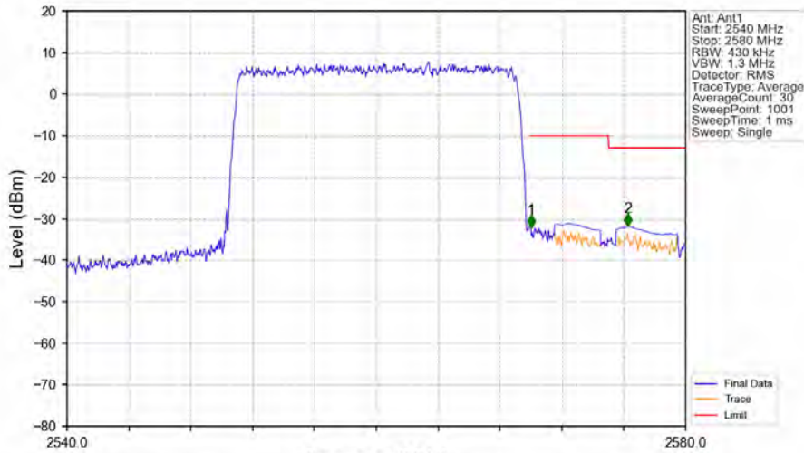
Band7_20MHz_QPSK_HCH_2560MHz_RB_100_0_NTNV
