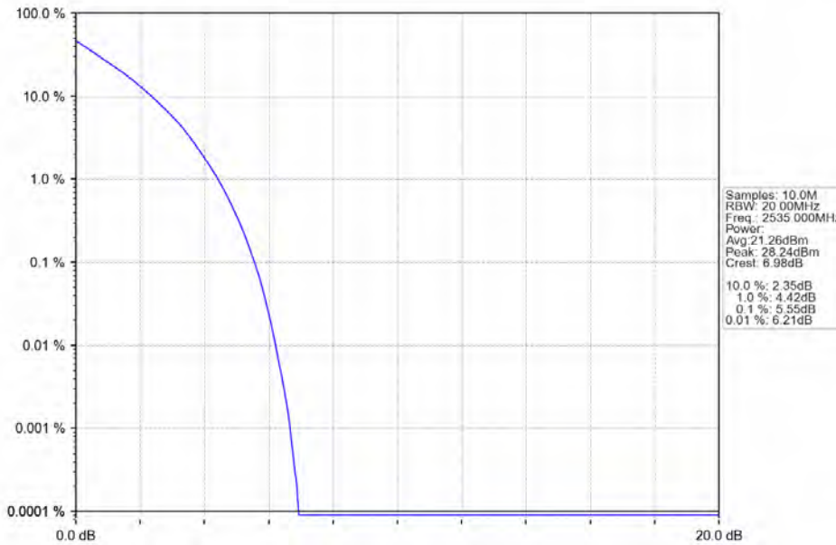
Band7_20MHz_QPSK_MCH_2535MHz_RB_100_0_NTNV
