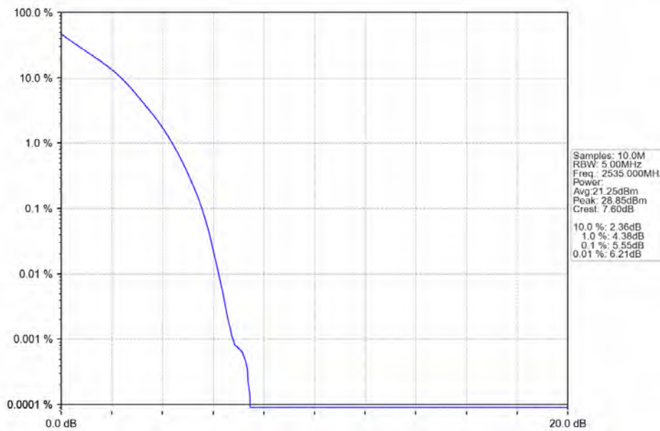
Band7_5MHz_QPSK_MCH_2535MHz_RB_25_0_NTNV
