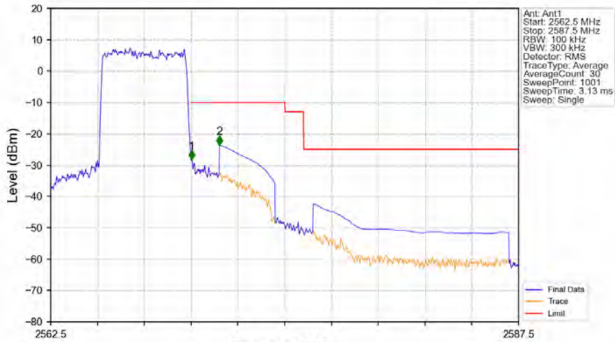
Band7_5MHz_QPSK_HCH_2567.5MHz_RB_25_0_NTNV
