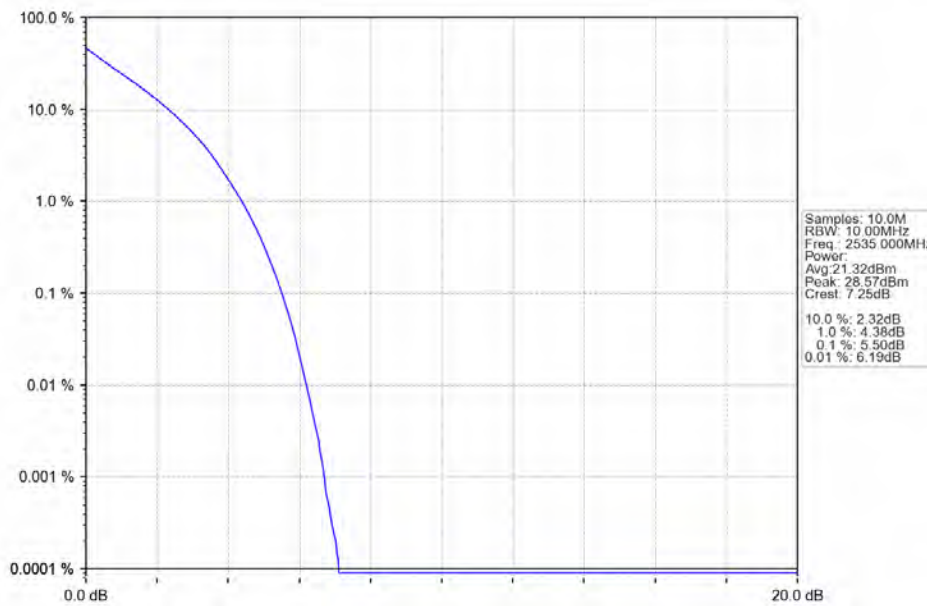
Band7_10MHz_QPSK_MCH_2535MHz_RB_50_0_NTNV
