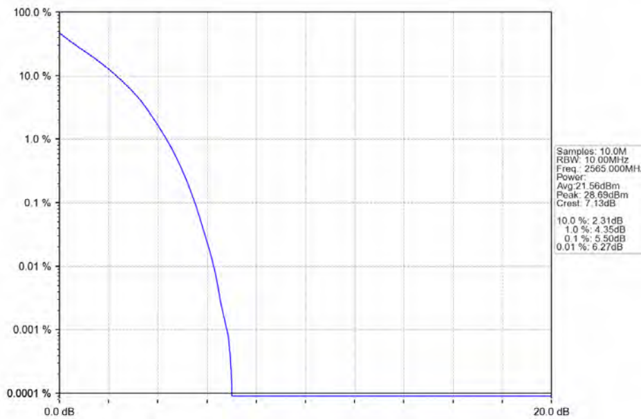
Band7_10MHz_QPSK_HCH_2565MHz_RB_50_0_NTV
