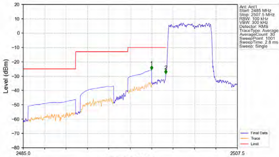
Band7_5MHz_QPSK_LCH_2502.5MHz_RB_25_0_NTNV
