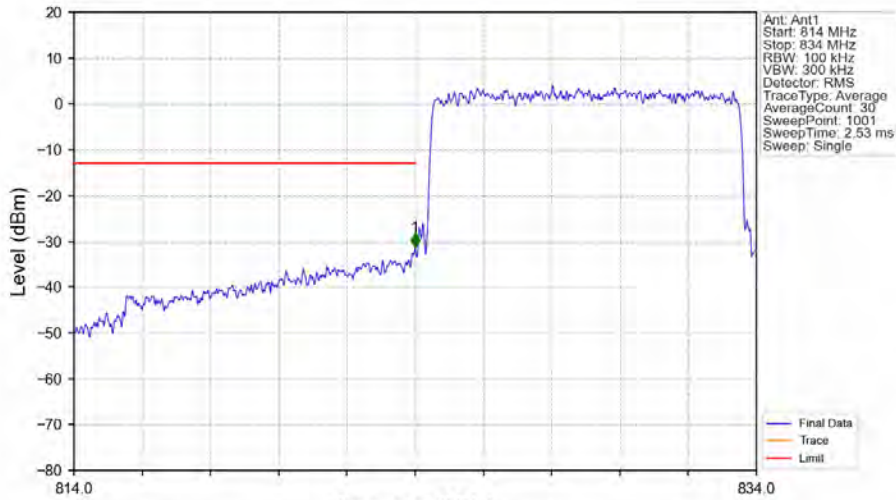
Band5_10MHz_QPSK_LCH_829MHz_RB_50_0_NTNV
