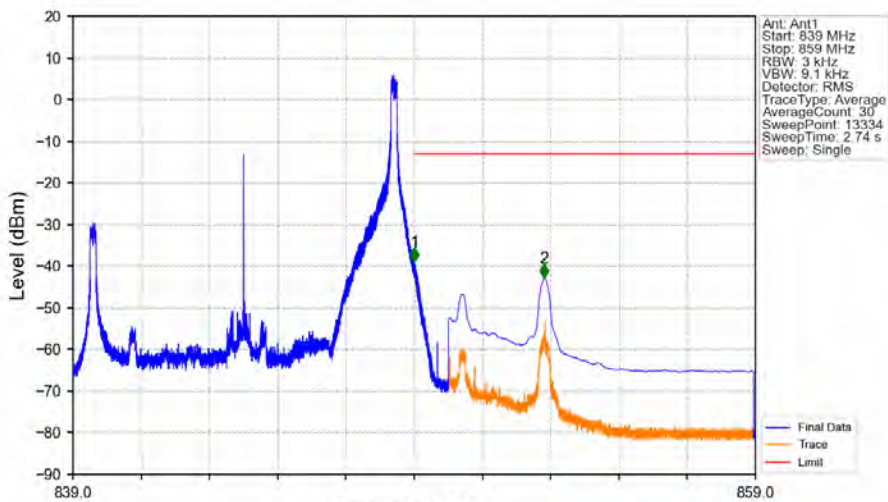
Band5_10MHz_QPSK_HCH_844MHz_RB_1_49_NTNV
