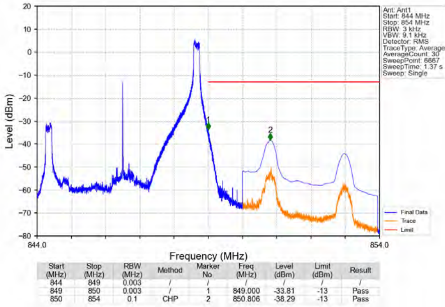
Band5_5MHz_QPSK_HCH_846.5MHz_RB_1_24_NTNV
