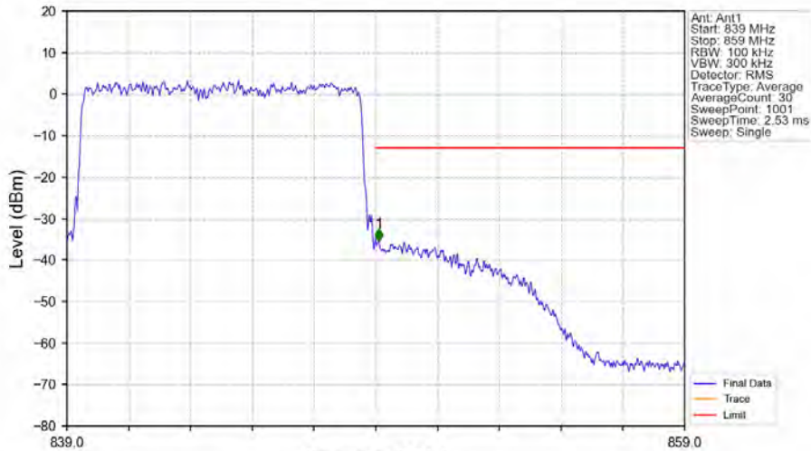
Band5_10MHz_QPSK_HCH_844MHz_RB_50_0_NTNV
