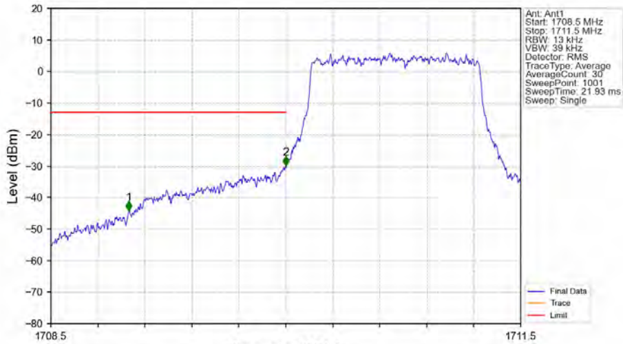
Band4 1.4MHz QPSK LCH 1710.7MHz RB 6 0 NTV
