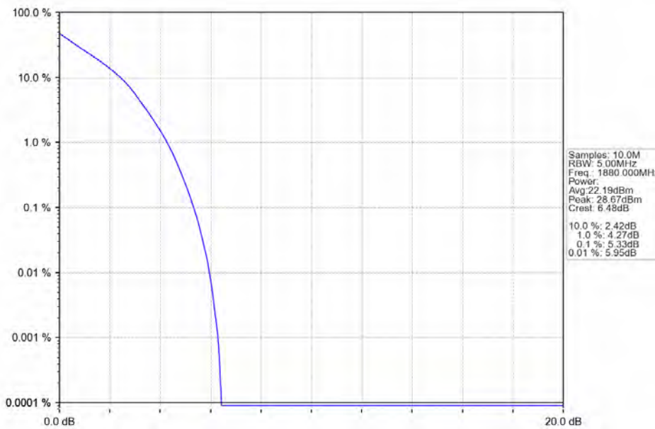
Band2_3MHz_QPSK_MCH_1880MHz_RB_15_0_NTNV
