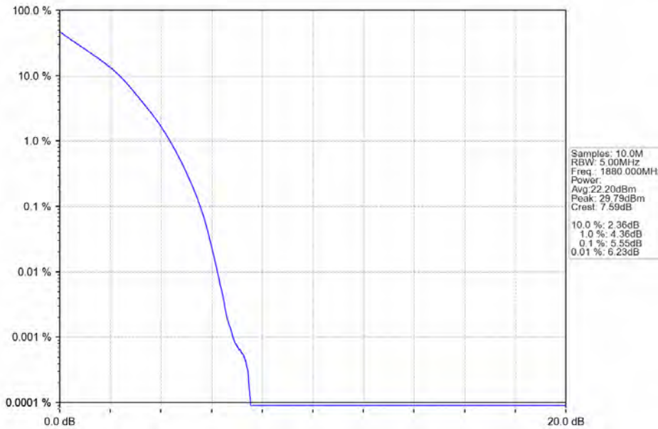
Band2_5MHz_QPSK_MCH_1880MHz_RB_25_0_NTNV
