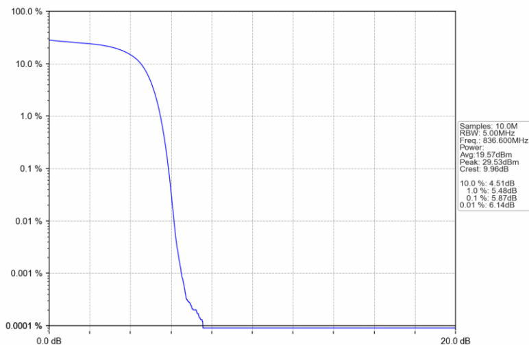
BandV_HSUPA_MCH_836.6MHz_Subtest 1_NTNV
