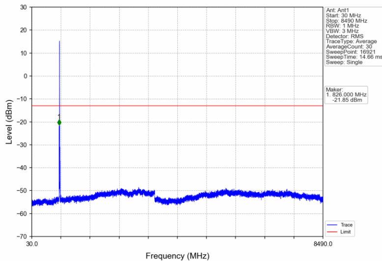
BandV_HSDPA_MCH_836.6MHz_Subtest 1_NTNV
