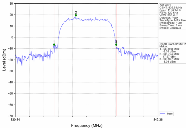
BandV_HSUPA_MCH_836.6MHz_Subtest 1_NTNV
