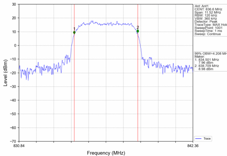
BandV_HSUPA_MCH_836.6MHz_Subtest 1_NTNV
