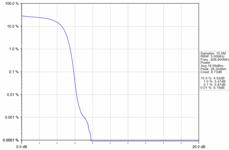
BandV_HSDPA_MCH_836.6MHz_Subtest 1_NTNV
