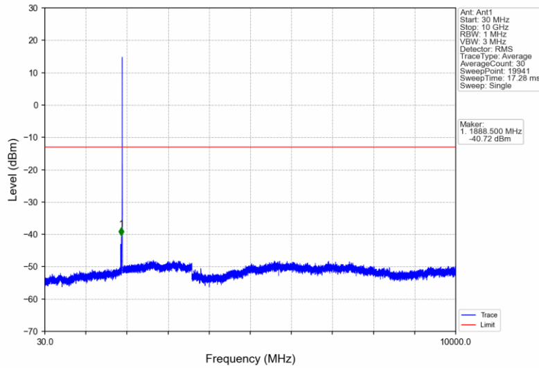
BandII_HSUPA_HCH_1907.6MHz_Subtest 1_NTNV
