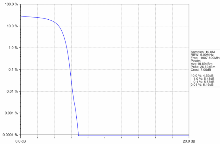
BandII_HSDPA_HCH_1907.6MHz_Subtest 1_NTNV
