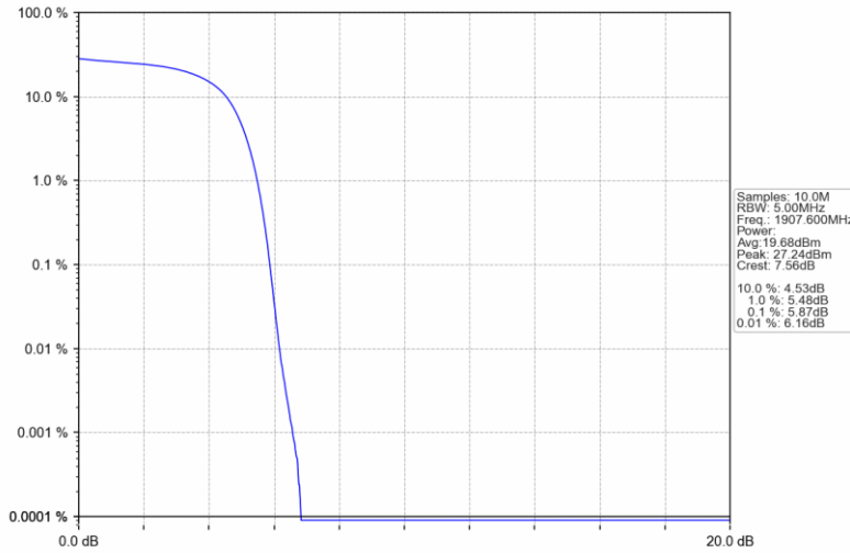
BandII_HSUPA_HCH_1907.6MHz_Subtest 1_NTNV
