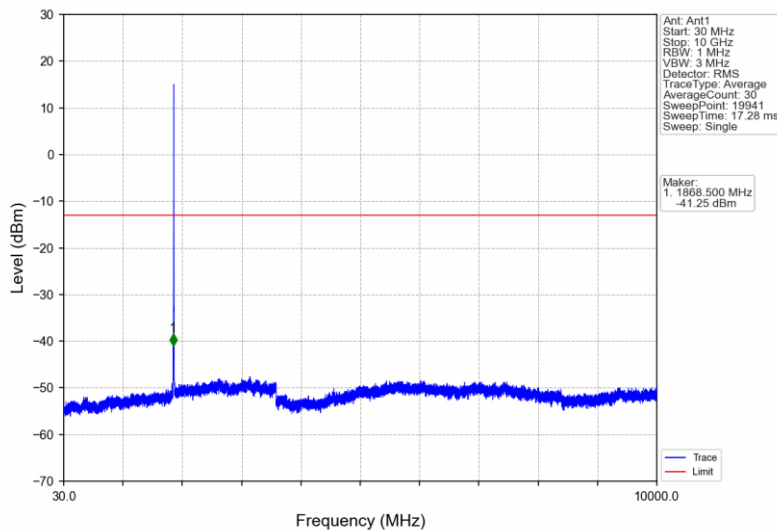
BandII_HSDPA_MCH_1880MHz_Subtest 1_NTNV
