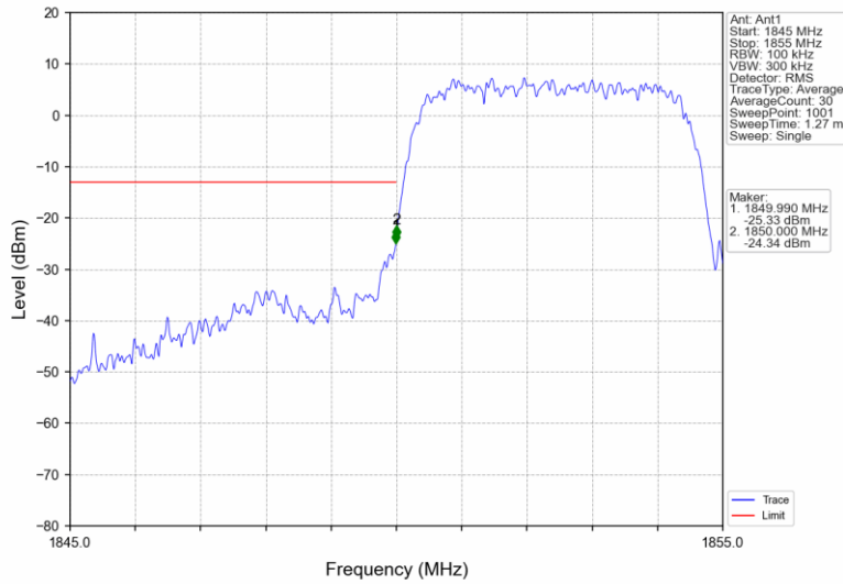
BandII_HSUPA_LCH_1852.4MHz_Subtest 1_NTNV
