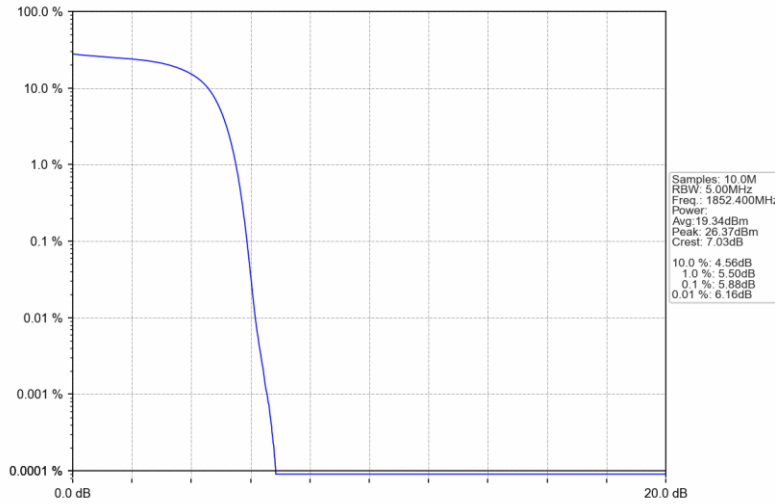
BandII_HSUPA_LCH_1852.4MHz_Subtest 1_NTNV
