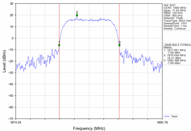
BandII_HSUPA_MCH_1880MHz_Subtest 1_NTNV
