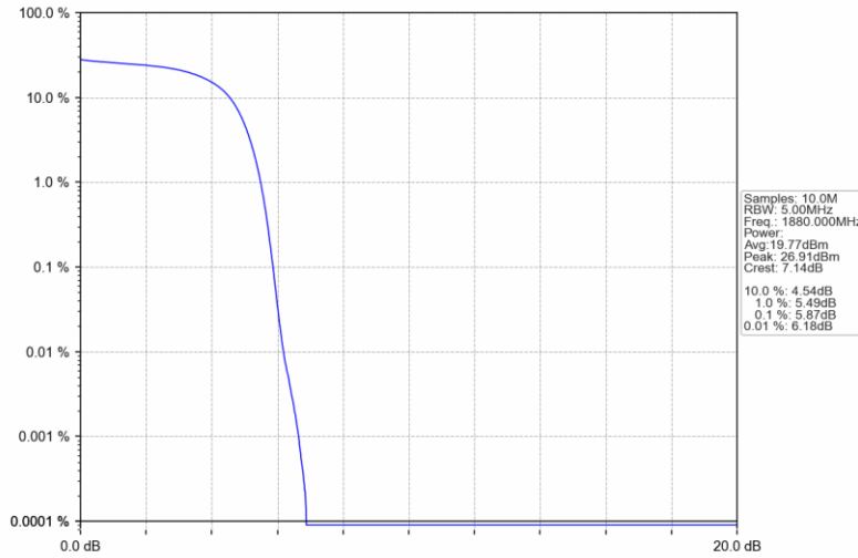
BandII_HSDPA_MCH_1880MHz_Subtest 1_NTNV
