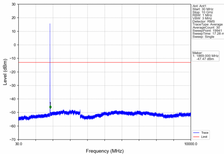
BandII_HSDPA_LCH_1852.4MHz_Subtest 1_NTNV
