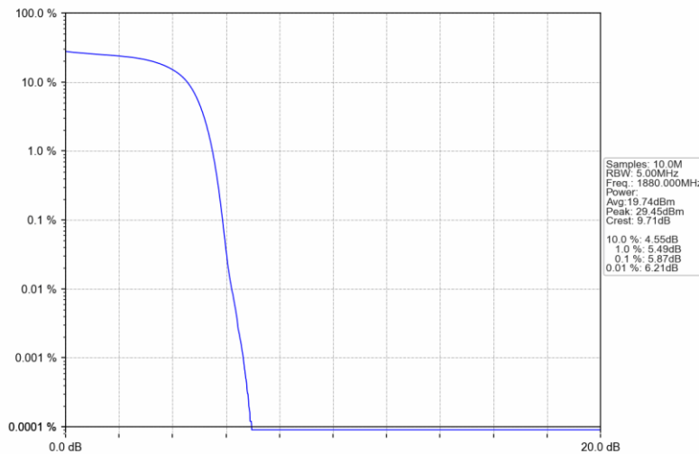
BandII_HSUPA_MCH_1880MHz_Subtest 1_NTNV
