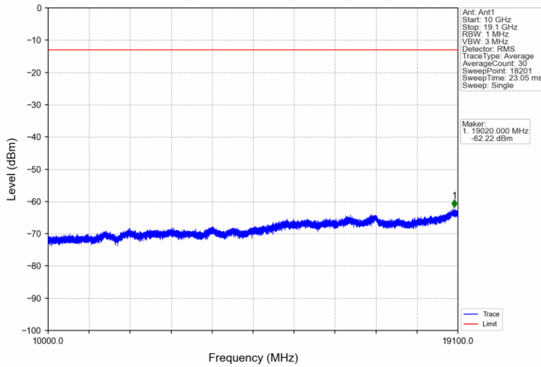
BandII_HSUPA_MCH_1880MHz_Subtest 1_NTNV
