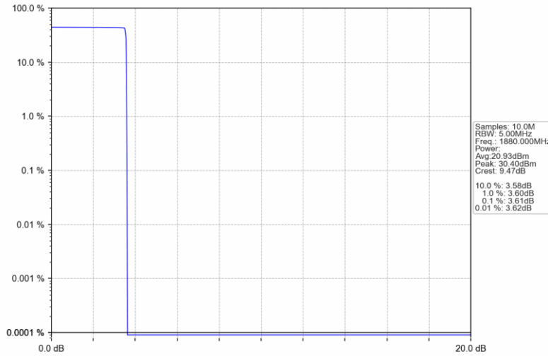
PCS1900_GPRS_MCH_1880MHz_4 TX Slots_NTNV
