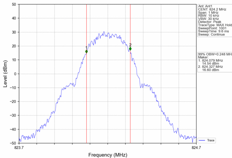
GSM850_GPRS_LCH_824.2MHz_1 TX Slot_NTNV
