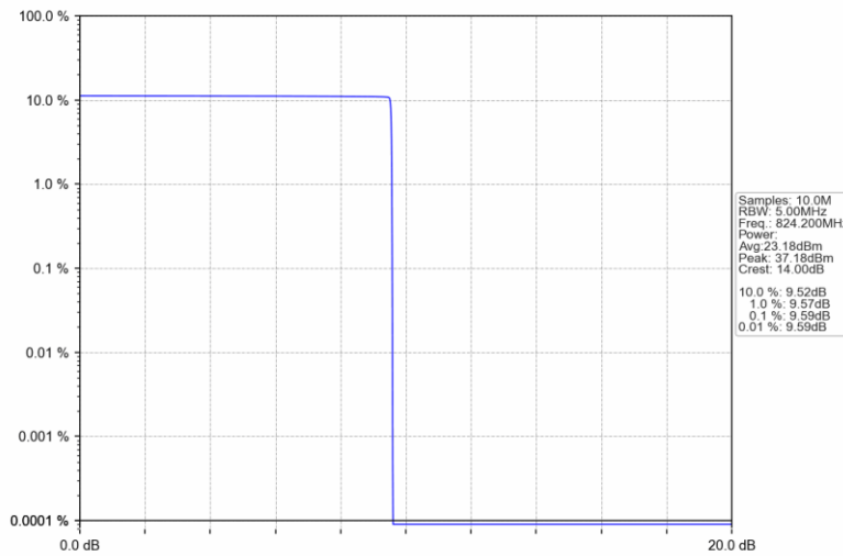
GSM850_GPRS_LCH_824.2MHz_4 TX Slots_NTNV
