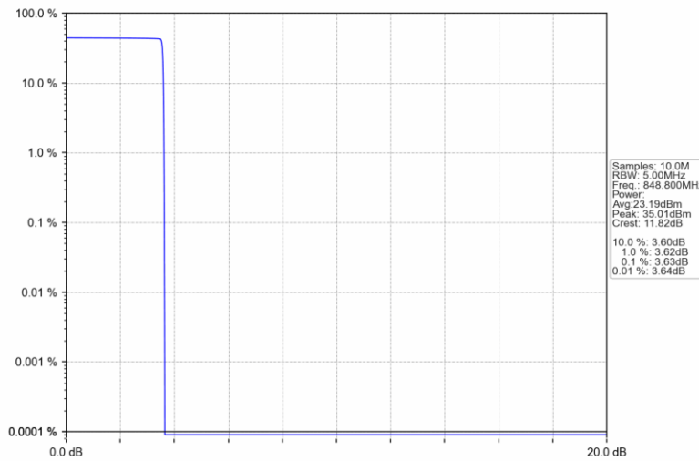
GSM850_GPRS_HCH_848.8MHz_4 TX Slots_NTNV
