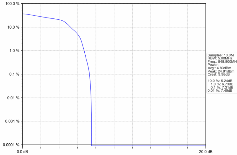
GSM850_EGPRS_HCH_848.8MHz_4 TX Slots_NTNV
