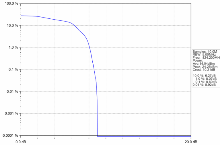
GSM850_EGPRS_LCH_824.2MHz_4 TX Slots_NTNV
