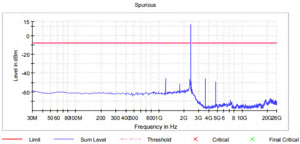
DH5_Ant1_2402_30~26500
