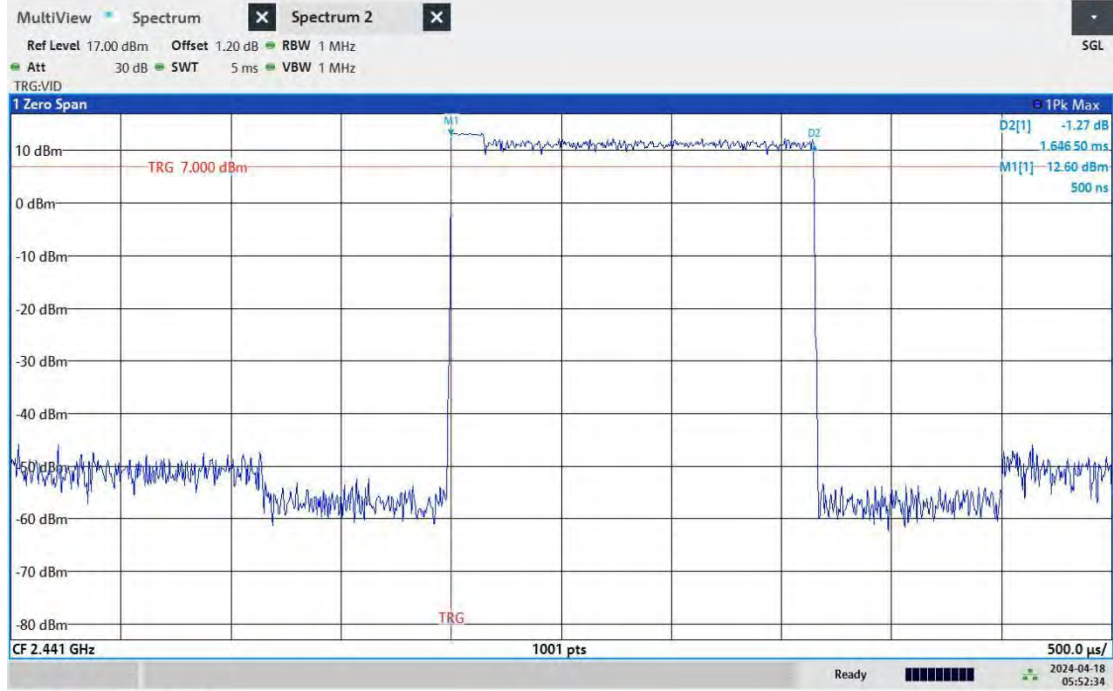
3DH3_Ant1_Hop
