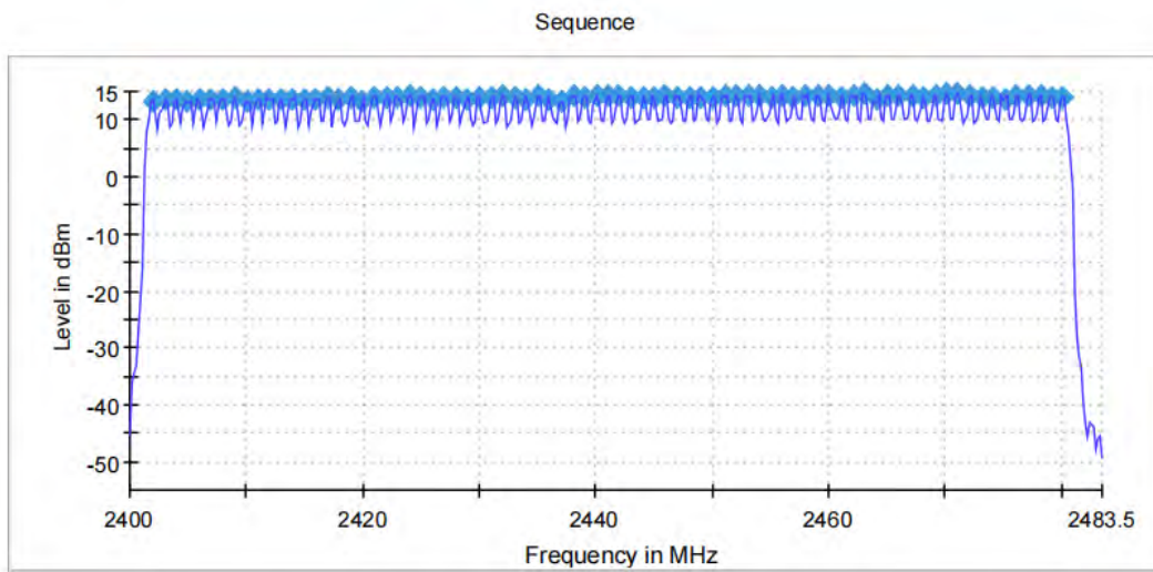
DH5_Ant1_Hop
