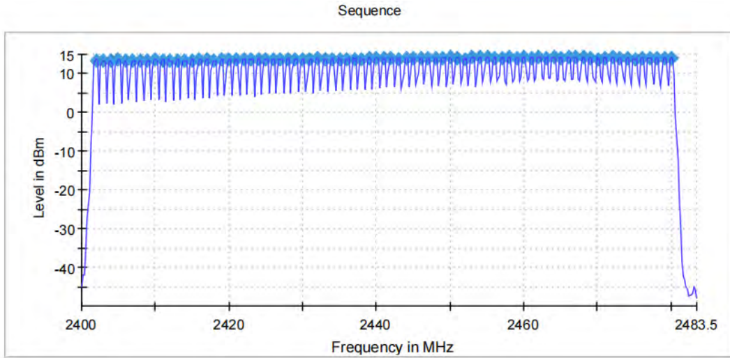
DH5_Ant1_Hop
