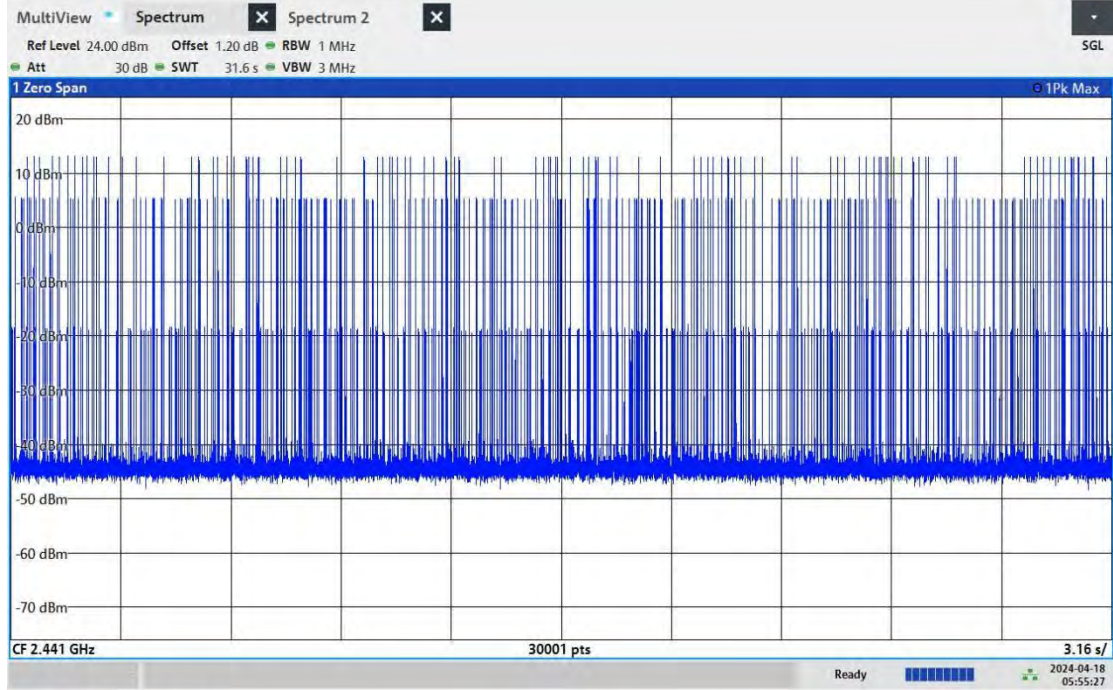
3DH5_Ant1_Hop
