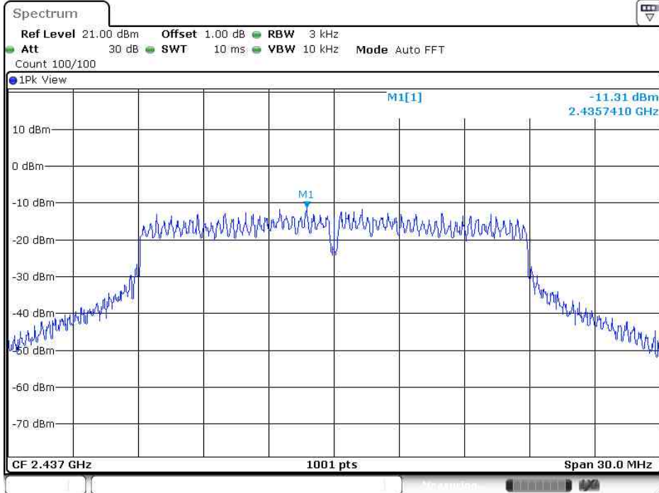
11N20SISO_Ant1_2437
