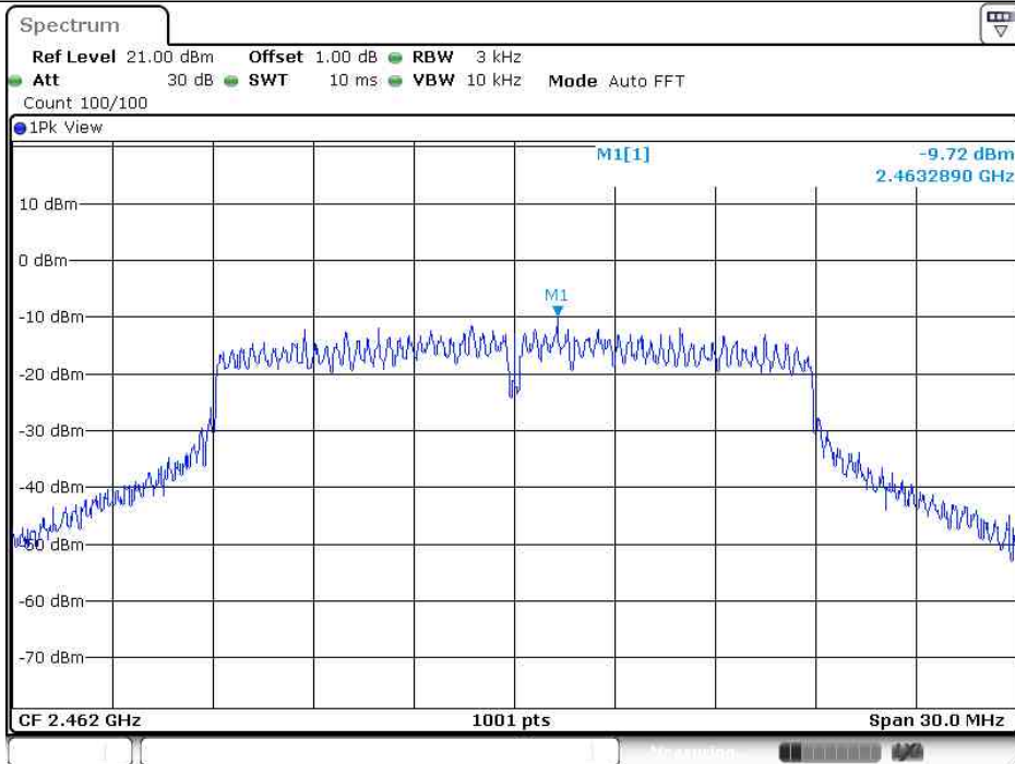
11N20SISO_Ant1_2462
