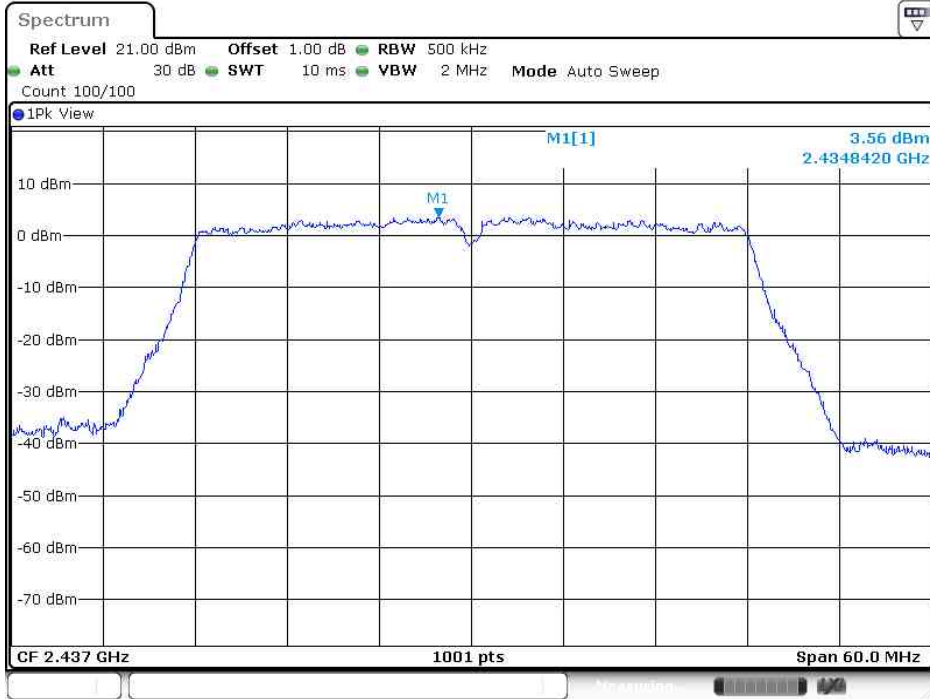
11N40SISO_Ant1_2437
