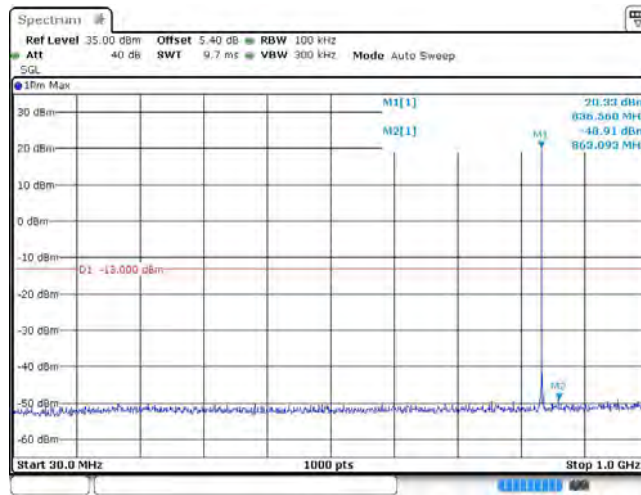
EGPRS850_190
