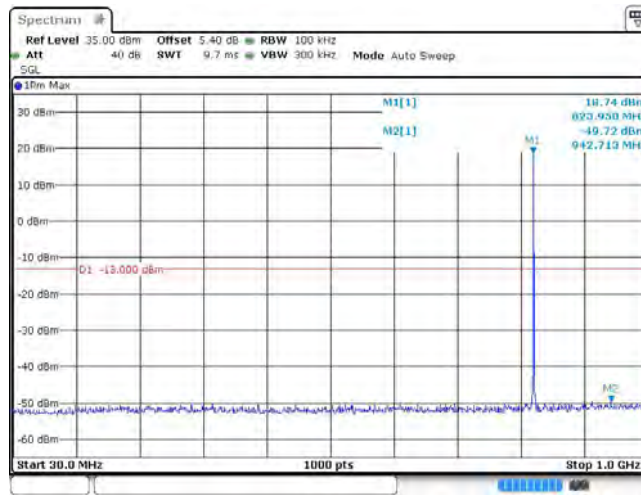
EGPRS850_128
