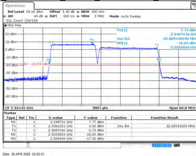
CA 7C 75RB+100RB_64QAM_20828+20999_75RB#0+100RB#0
