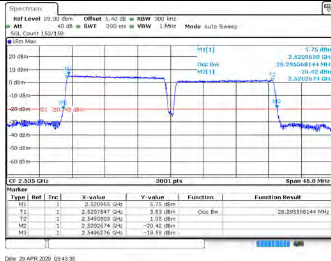
CA 7C 75RB+75RB QPSK 21225+21375 75RB#0+75RB#0
