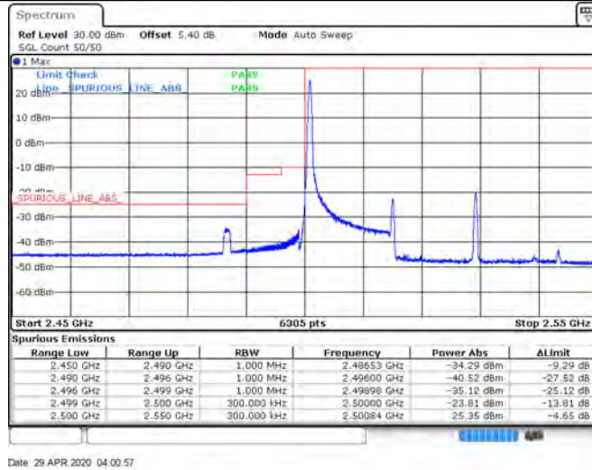
CA_7C_75RB+75RB_16QAM_20825+20975_75RB#0+75RB#0
