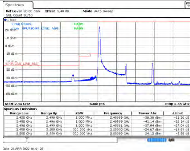
CA 7C_75RB+75RB_64QAM_20825+20975_75RB#0+75RB#0
