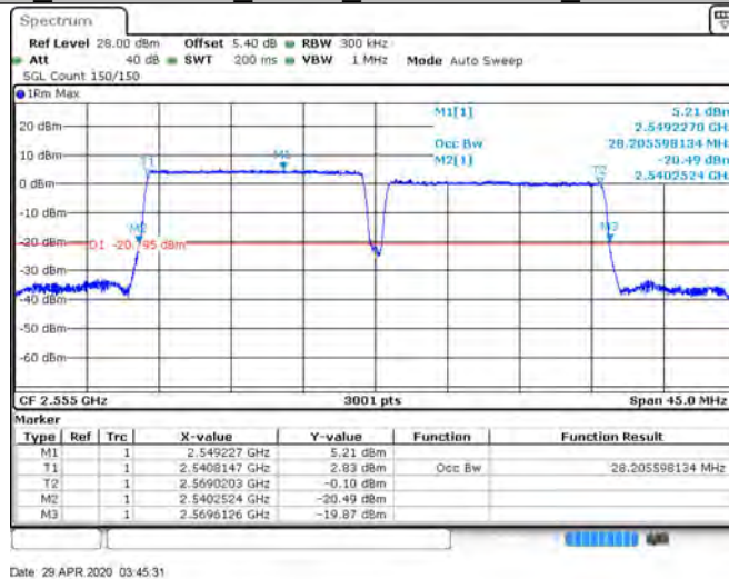
CA 7C 75RB+75RB 16QAM 20825+20975 75RB#0+75RB#0
