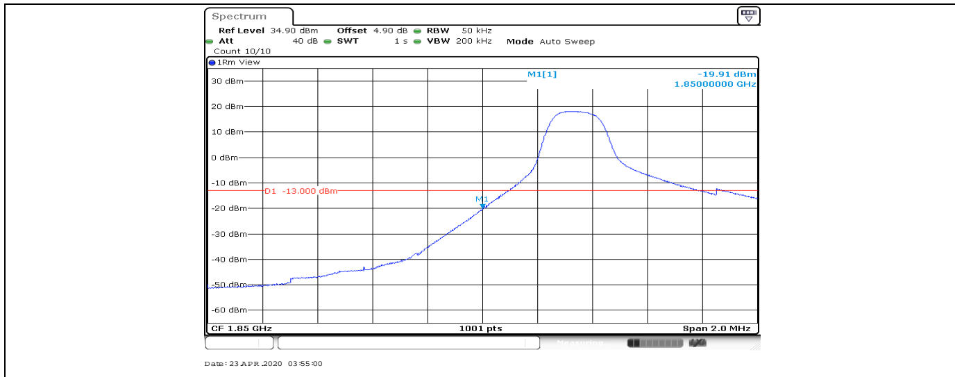
Band2-5MHz-QPSK-18625-25RB#0
