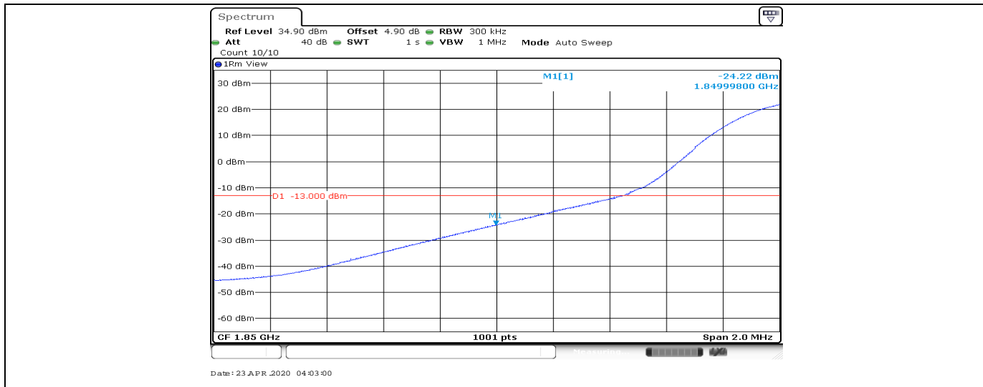
Band2-20MHz-QPSK-18700-100RB#0
