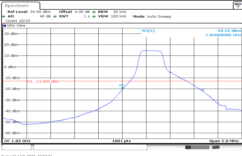
Band2-3MHz-16QAM-18615-15RB#0
