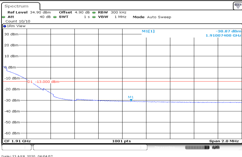
Band2-20MHz-64QAM-18700-1RB#0
