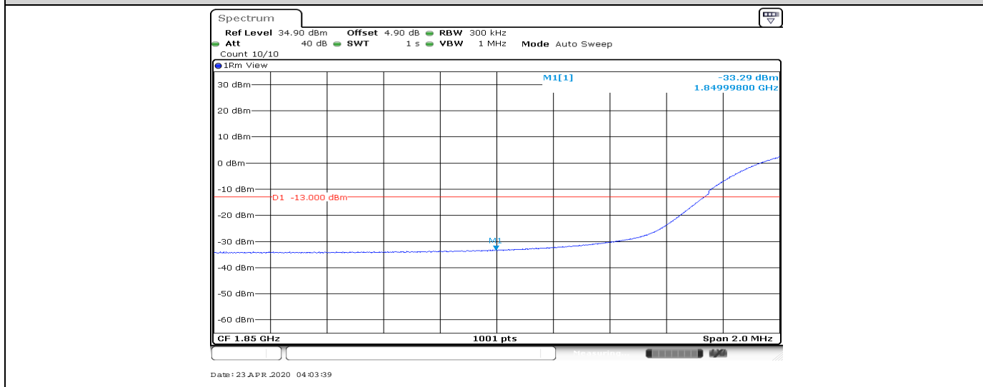
Band2-20MHz-QPSK-19100-1RB#99
