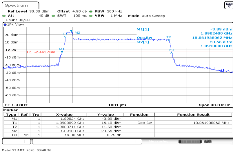
Band2-20MHz-64QAM-18700-100RB#0-18.062
