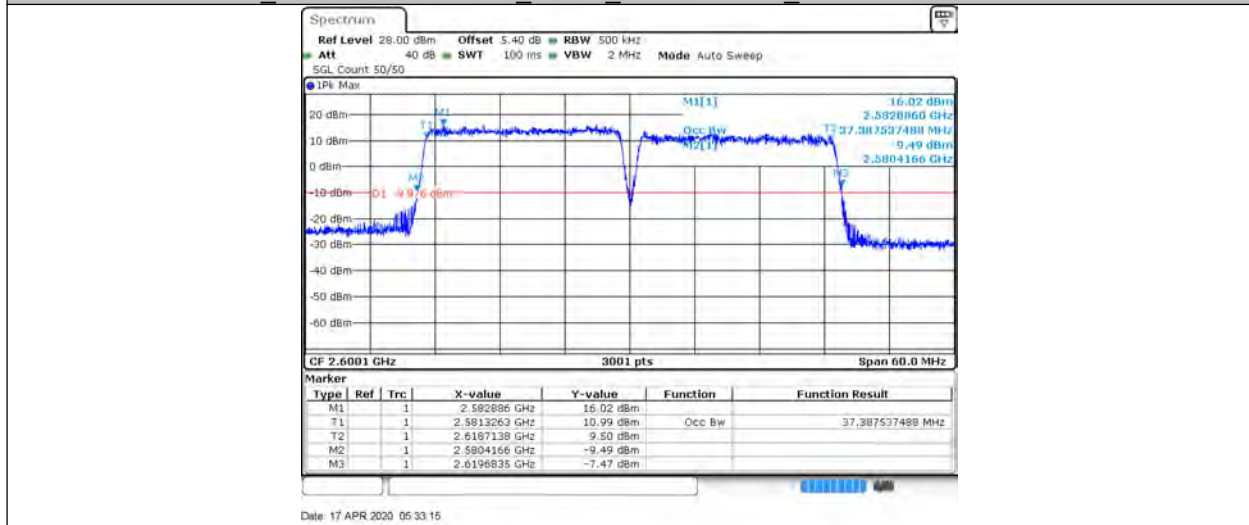
CA 38C 20MHz+20MHz 16QAM 37850+38048 100RB#0+100RB#0
