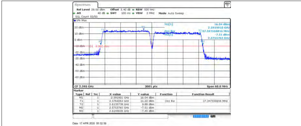
CA 38C 20MHz+20MHz QPSK 37952+38150 100RB#0+100RB#0
