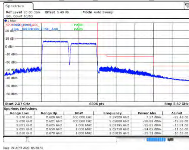
CA 38C 100RB+100RB QPSK 37850+38048 1RB#0+0RB#0
