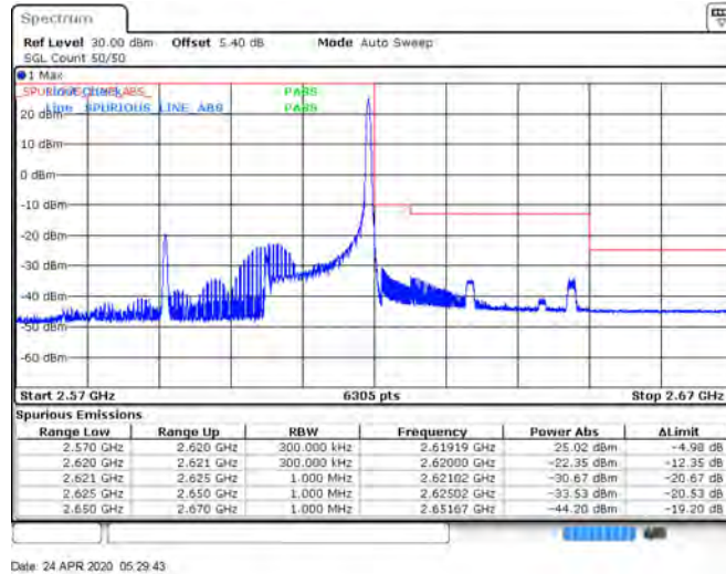
CA 38C 75RB+75RB 64QAM 38025+38175 75RB#0+75RB#0
