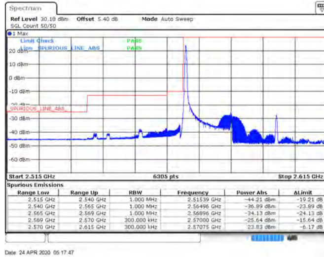
CA 38C 75RB+75RB 64QAM 37825+37975 75RB#0+75RB#0
