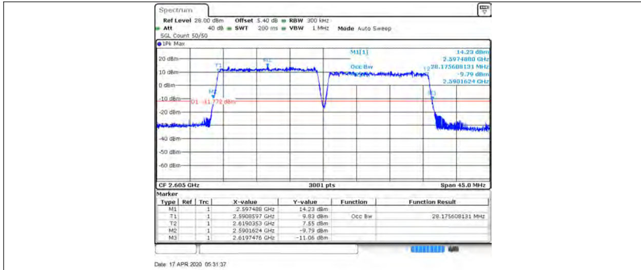
CA_38C 20MHz+20MHz QPSK 37850+38048 100RB#0+100RB#0
