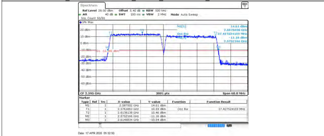
CA 38C 20MHz+20MHz 16QAM 37952+38150 100RB#0+100RB#0
