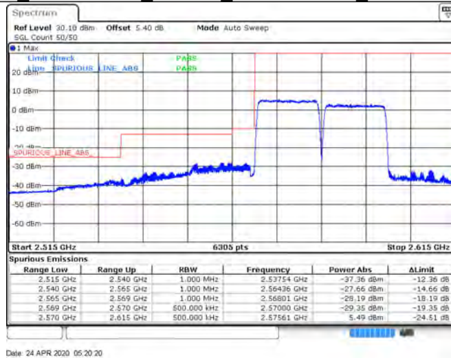
CA 38C 75RB+75RB 16QAM 37825+37975 75RB#0+75RB#0
