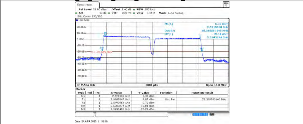
CA 7C 15+15 QPSK 21225+21375_75RB#0+75RB#0
