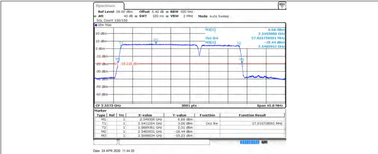
CA_7C_20+10_16QAM_20850+20994_100RB#0+50RB#0
