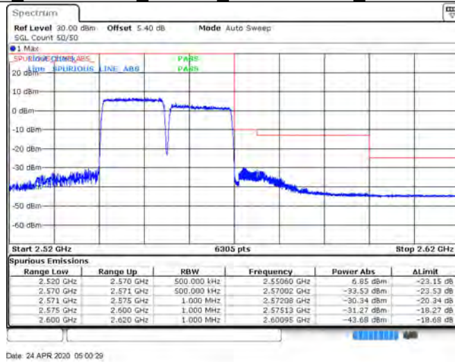
CA 7C 75RB+75RB 64QAM 208225RB+100RB975 1RB#0+0RB#0
