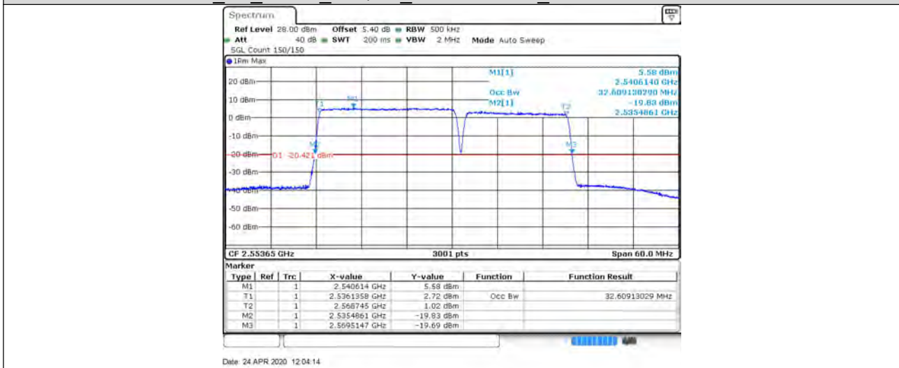
CA_7C_20+20_QPSK_20850+21048_100RB#0+100RB#0
