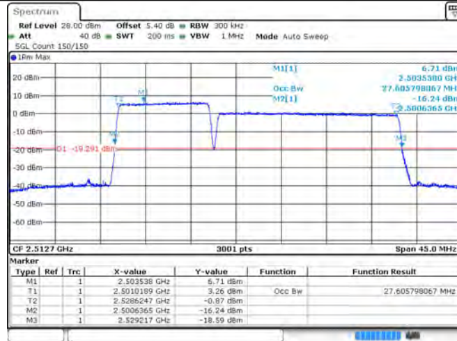
CA_7C_10+20_QPSK_20805+20949_50RB#0+100RB#0
