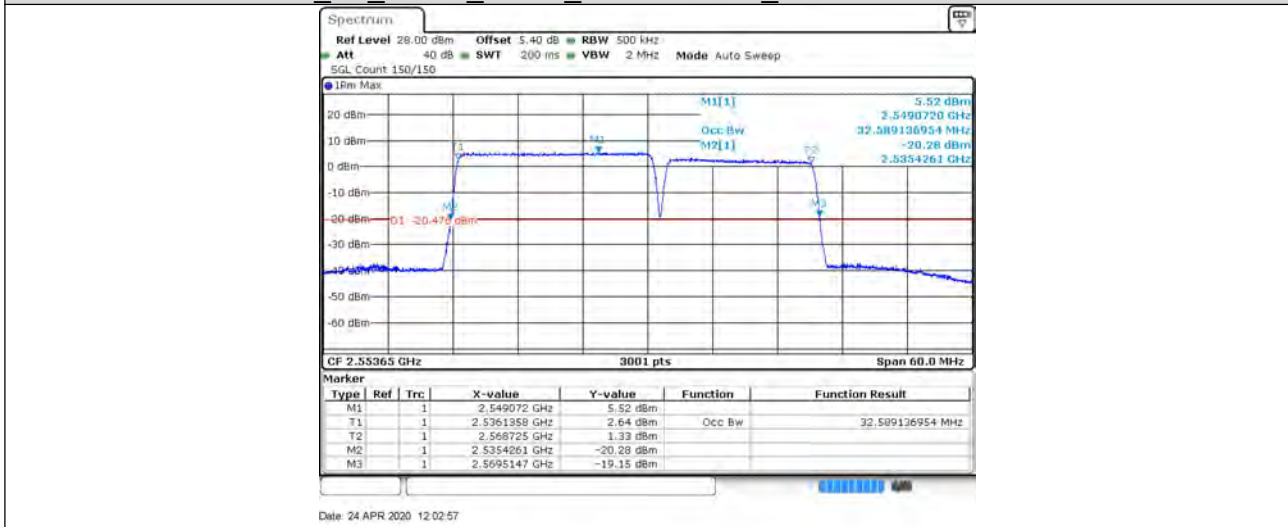
CA 7C 20+15 16QAM 20850+21021_100RB#0+75RB#0
