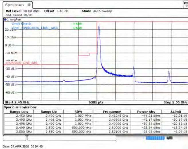
CA_7C_100RB+100RB_QPSK_20850+21048_100RB#0+100RB#0
