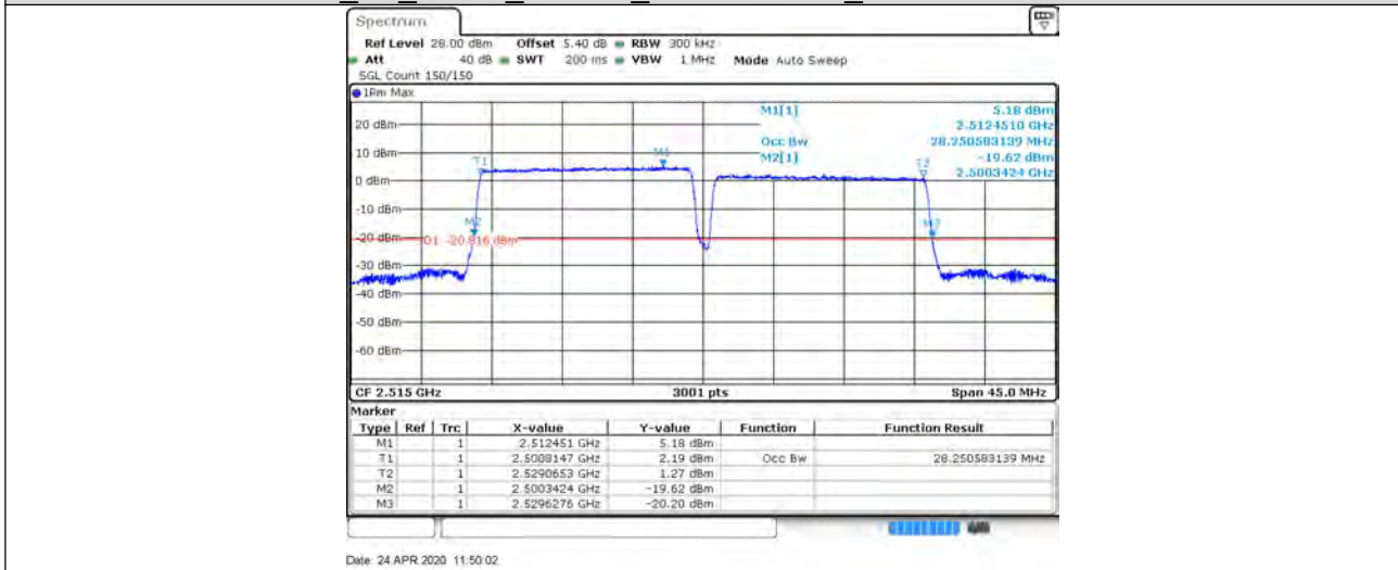
CA 7C_15+15_16QAM_21025+21175_75RB#0+75RB#0
