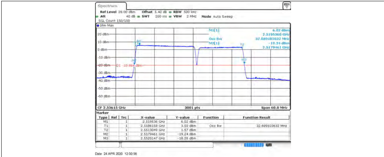
CA 7C 20+15 QPSK 21201+21372_100RB#0+75RB#0
