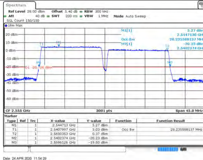
CA 7C_15+20_QPSK_20828+20999_75RB#0+100RB#0
