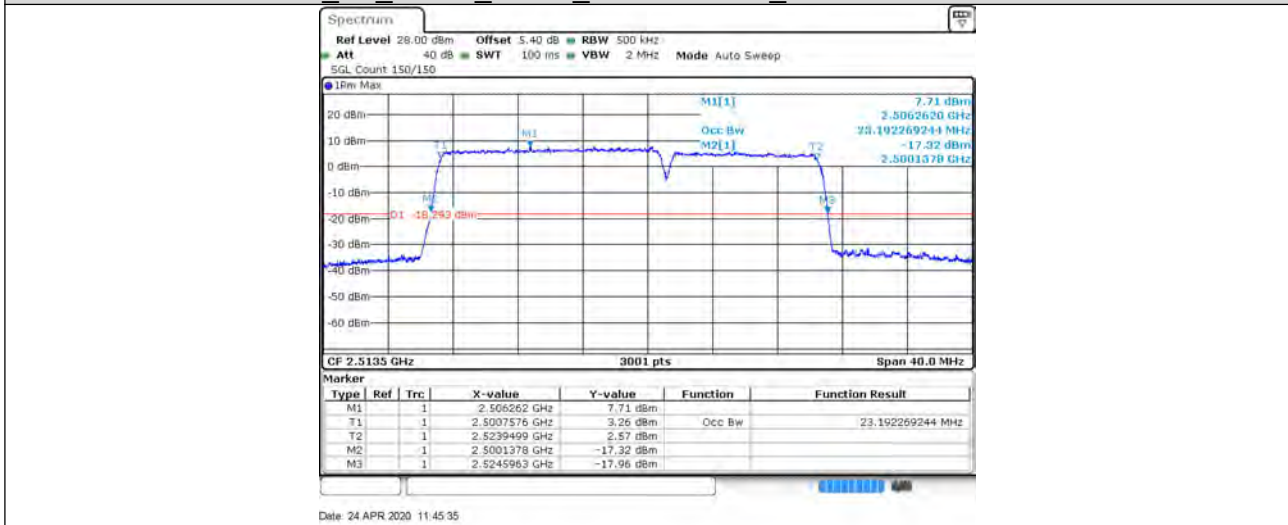
CA 7C 15+10 QPSK 21051+21171_75RB#0+50RB#0
