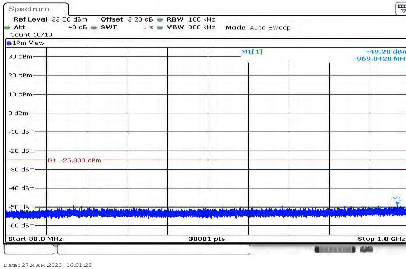
Band38-20MHz-QPSK-38150-1RB#0-Range2:1000~30000MHz
