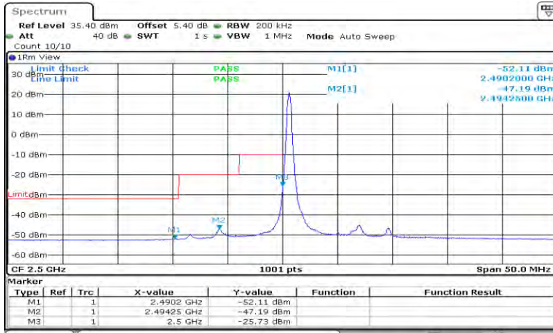
Band7-10MHz-QPSK-20800-50RB#0
