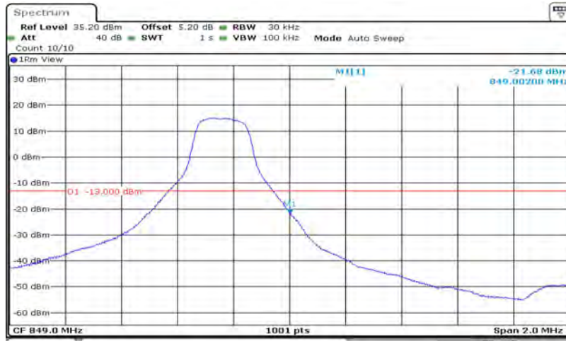
Band5-3MHz-QPSK-20635-15RB#0
