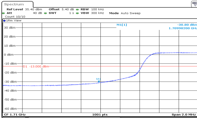
Band4-10MHz-QPSK-20000-50RB#0
